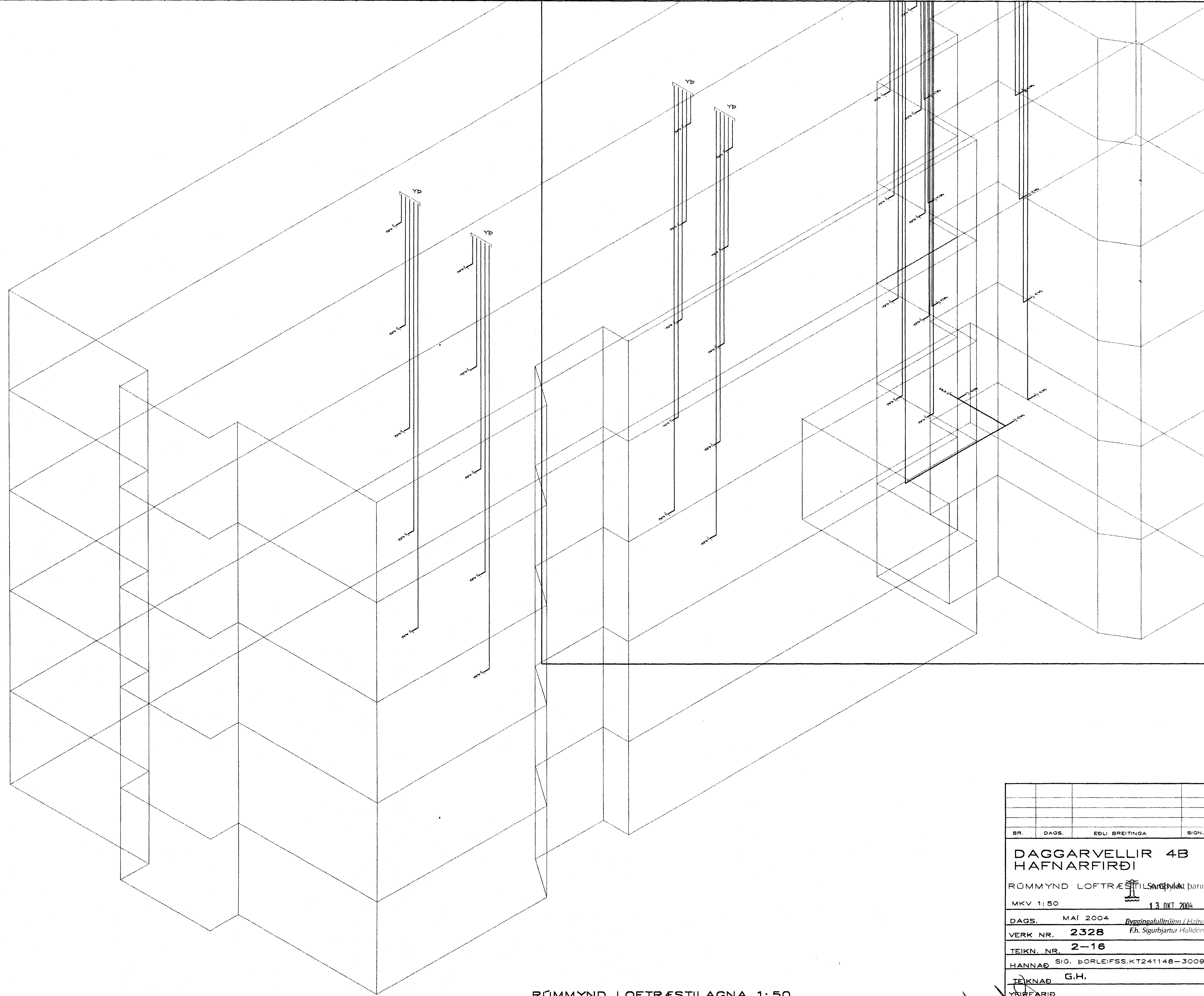
RÜMMYND LOFTRÆSTILAGNA 1:50
