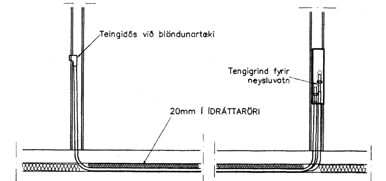
TENGING NEYSLUVATNSLAGNA 1:20
