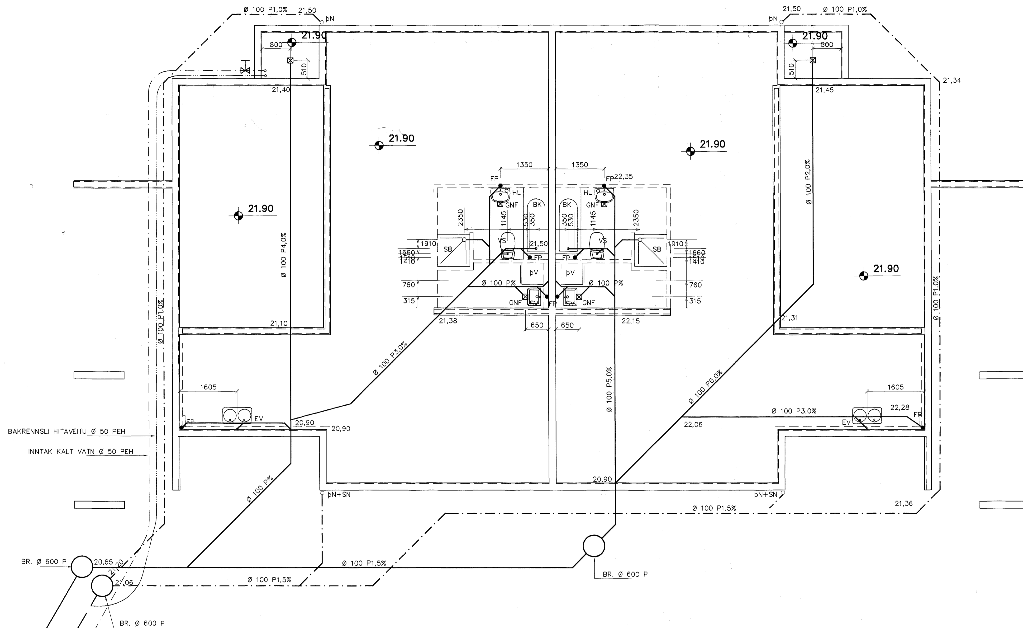
GRUNNMYND 1:50
