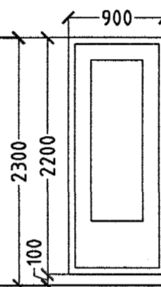
1. STK. STOFA. HURÐ OPNAST VINSTRI ÚT. 2. STK. STOFA. HURÐ OPNAST HÆGRI ÚT.
