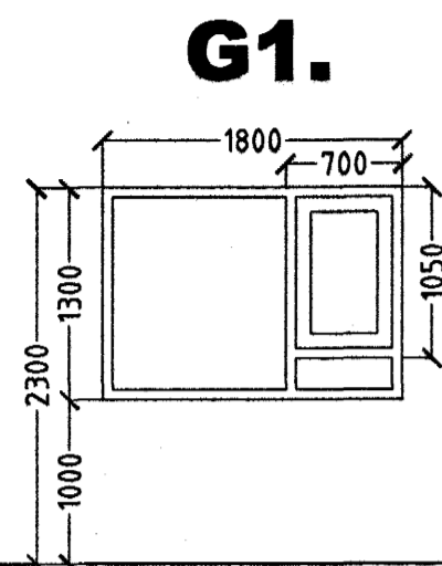
G1. 10. STK. HERB./HJÓN. BJÖRGUNAROP.
