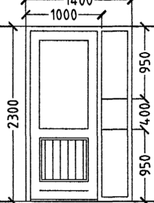
1. STK. ANDDYRI. HURÐ OPNAST HÆGRI INN.
