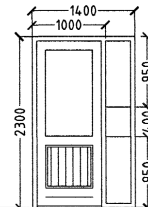
1. STK. ANDDYRI. HURÐ OPNAST HÆGRI INN.
