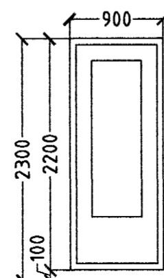
1. STK. STOFA. HURÐ OPNAST VINSTRI ÚT. 2. STK. STOFA. HURÐ OPNAST HÆGRI ÚT.
