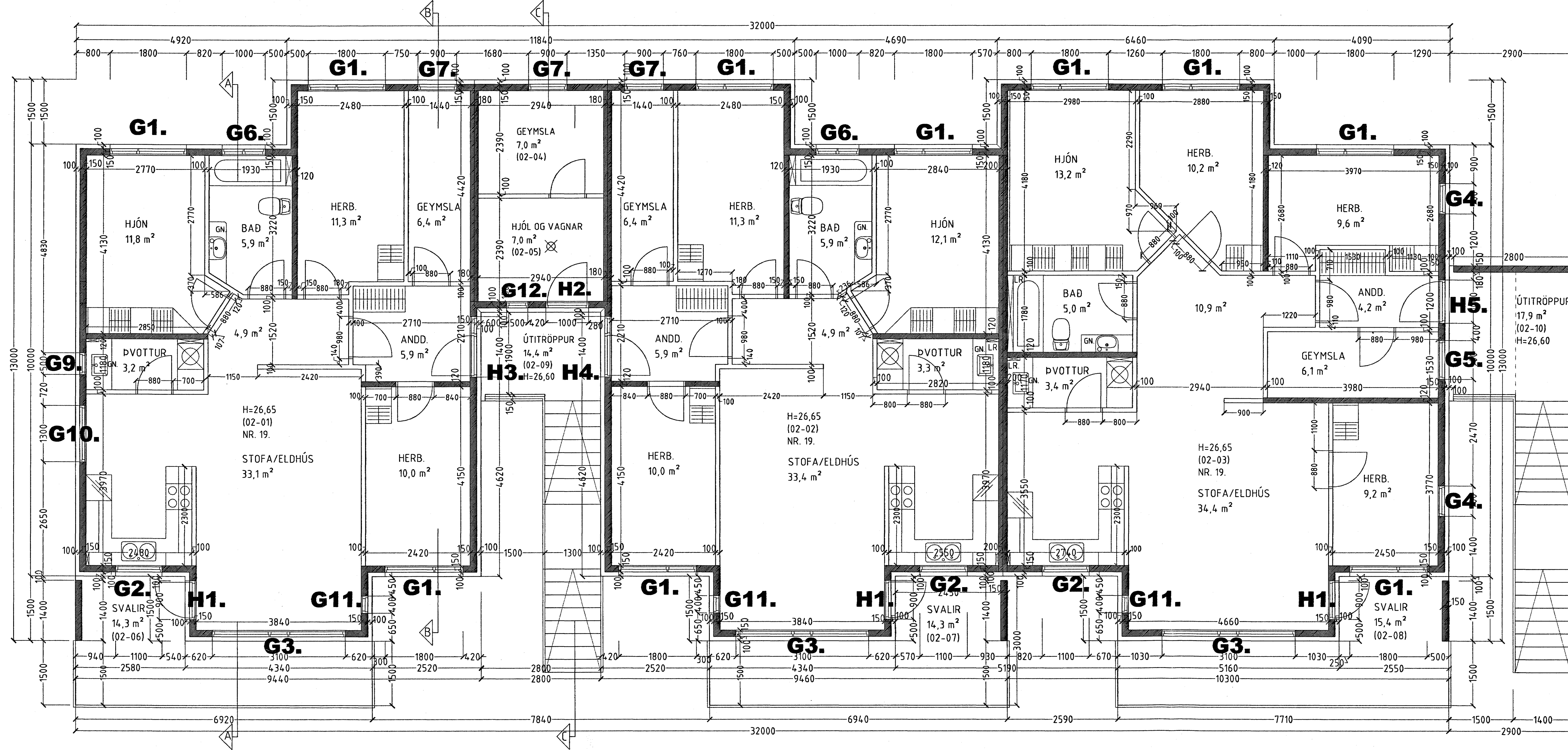
GRUNNMYND 2. HÆÐ MKV. 1:50.
