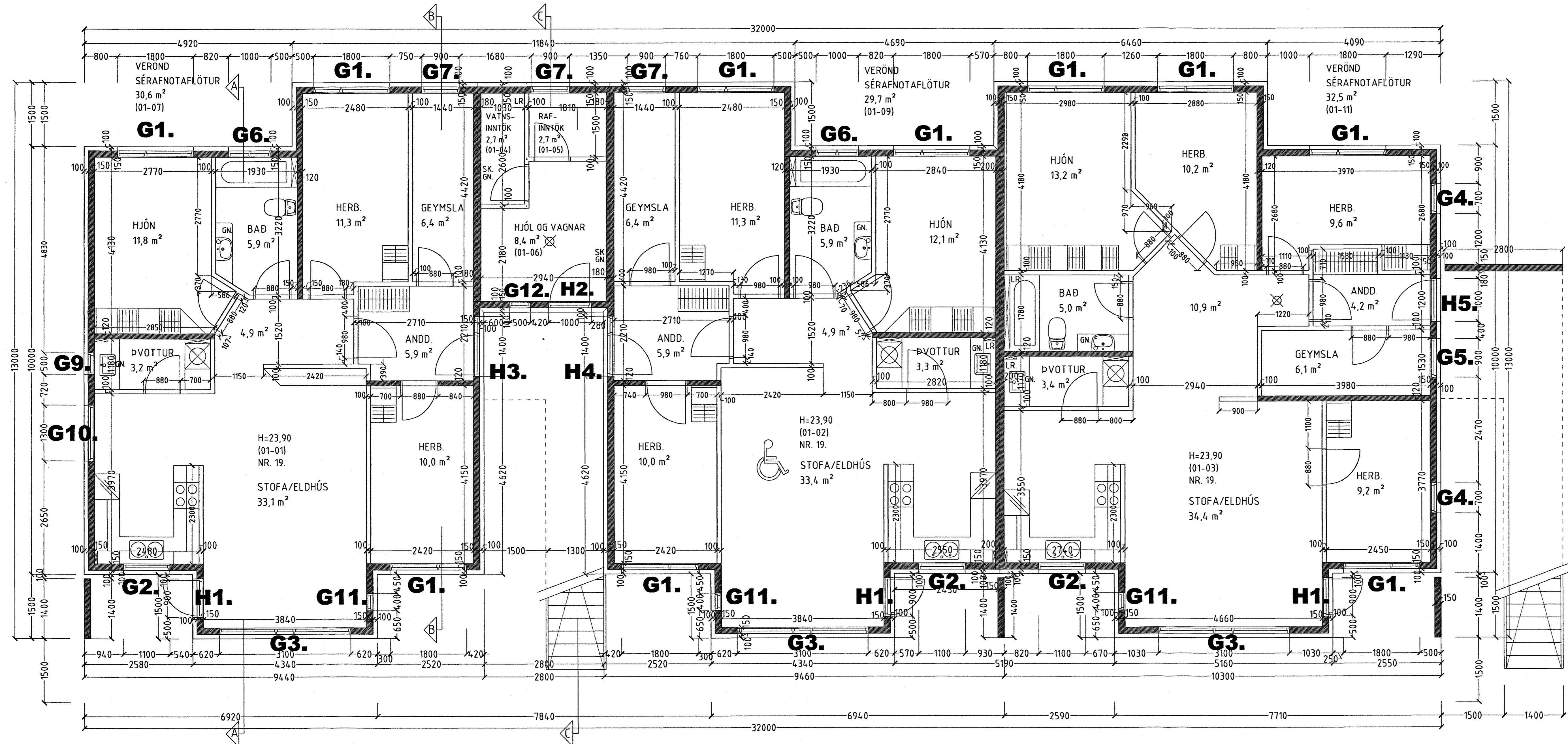
GRUNNMYND 1. HÆÐ MKV. 1:50.
