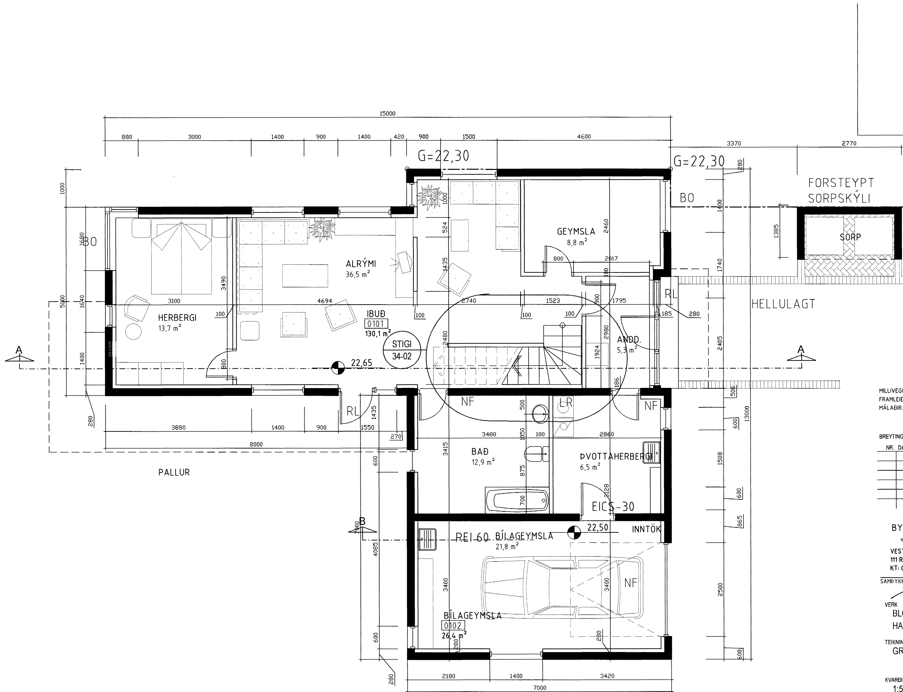
GRUNNMYND 1.HÆÐ 1:50
