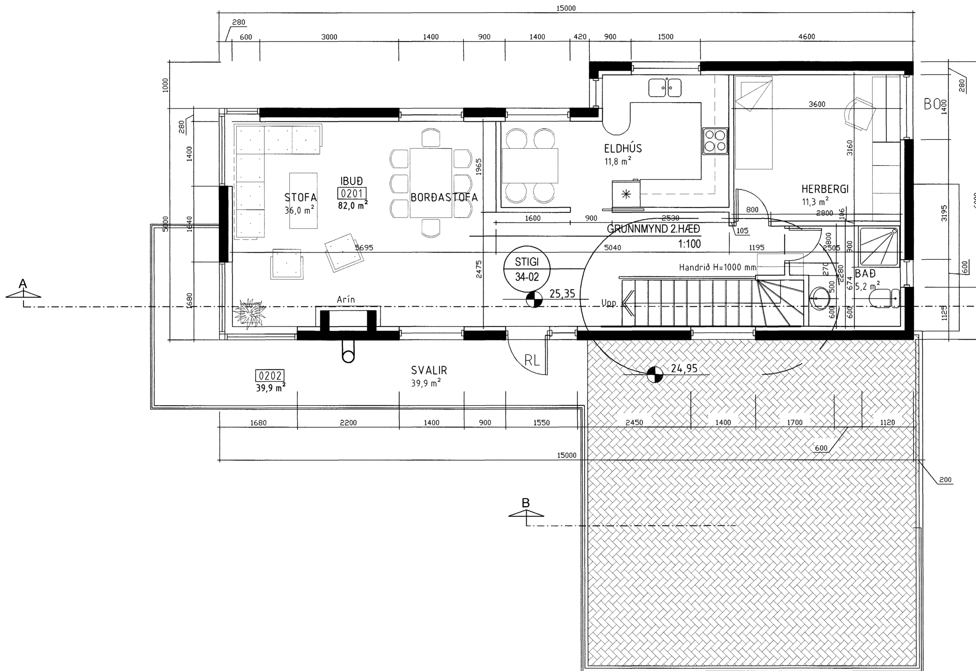
GRUNNMYND 1.HÆÐ 1:50
