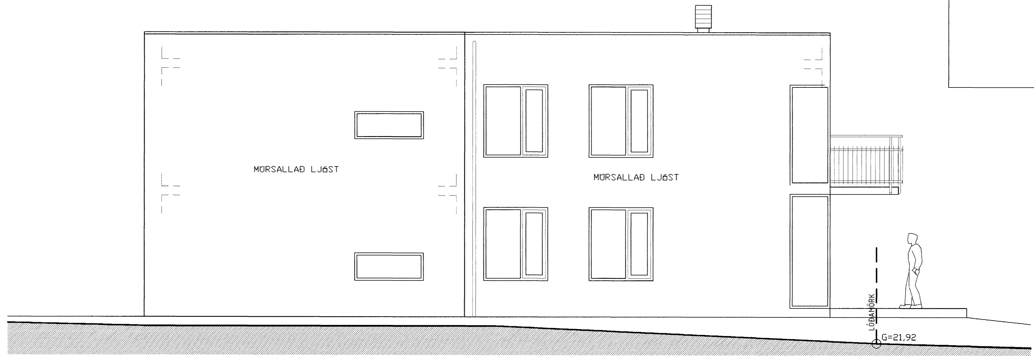
ÚTLIT NORÐUR 1:50
