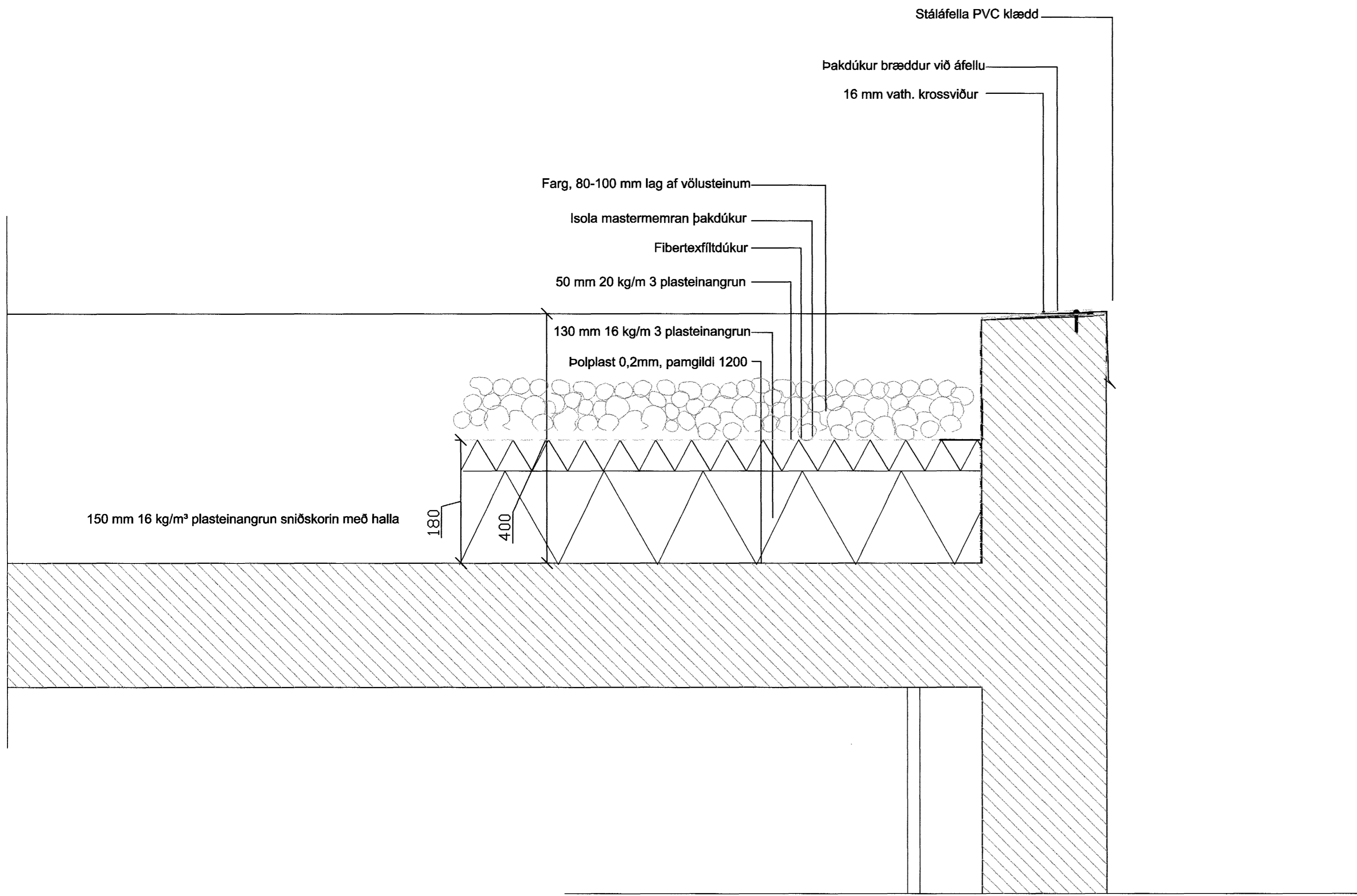
ÞAKDEILIR EFRA ÞAK 1:5
