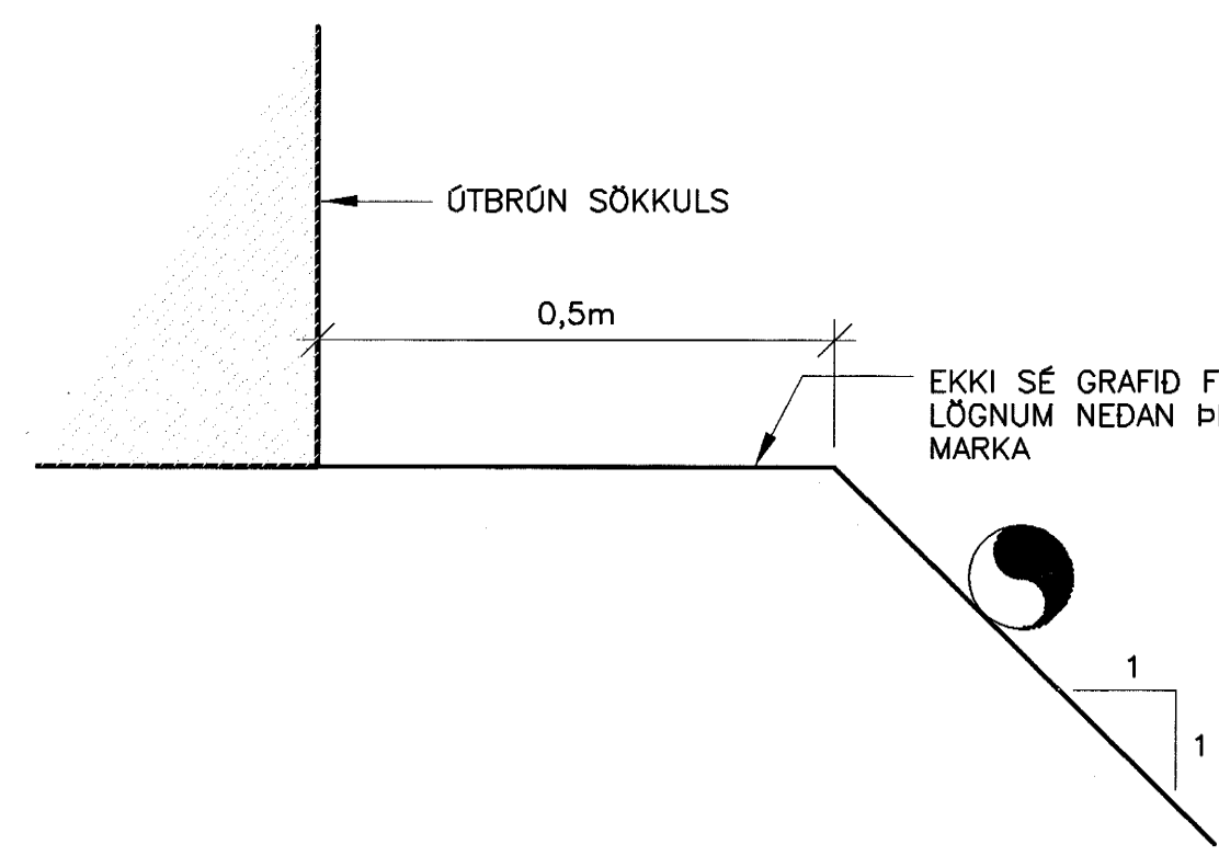
LEGA LAGNA VÍD HÚS 1:10
