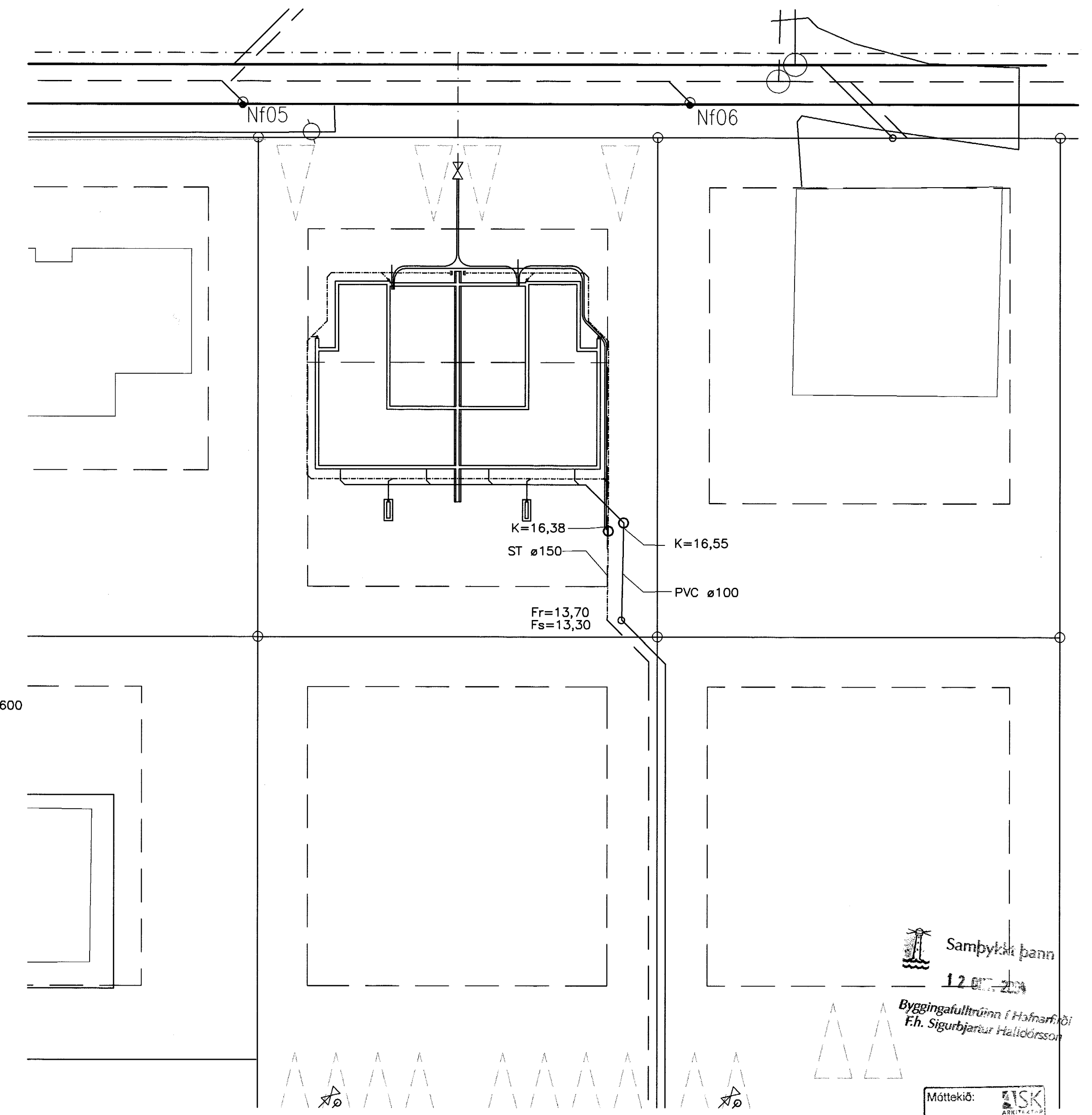
AFSTÖÐUMÝND. 1:200
