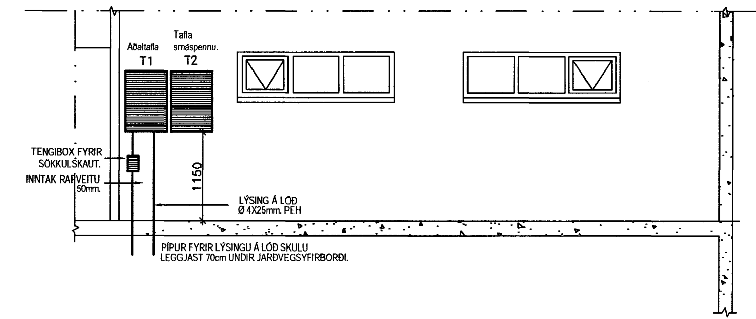
SNID A-A
