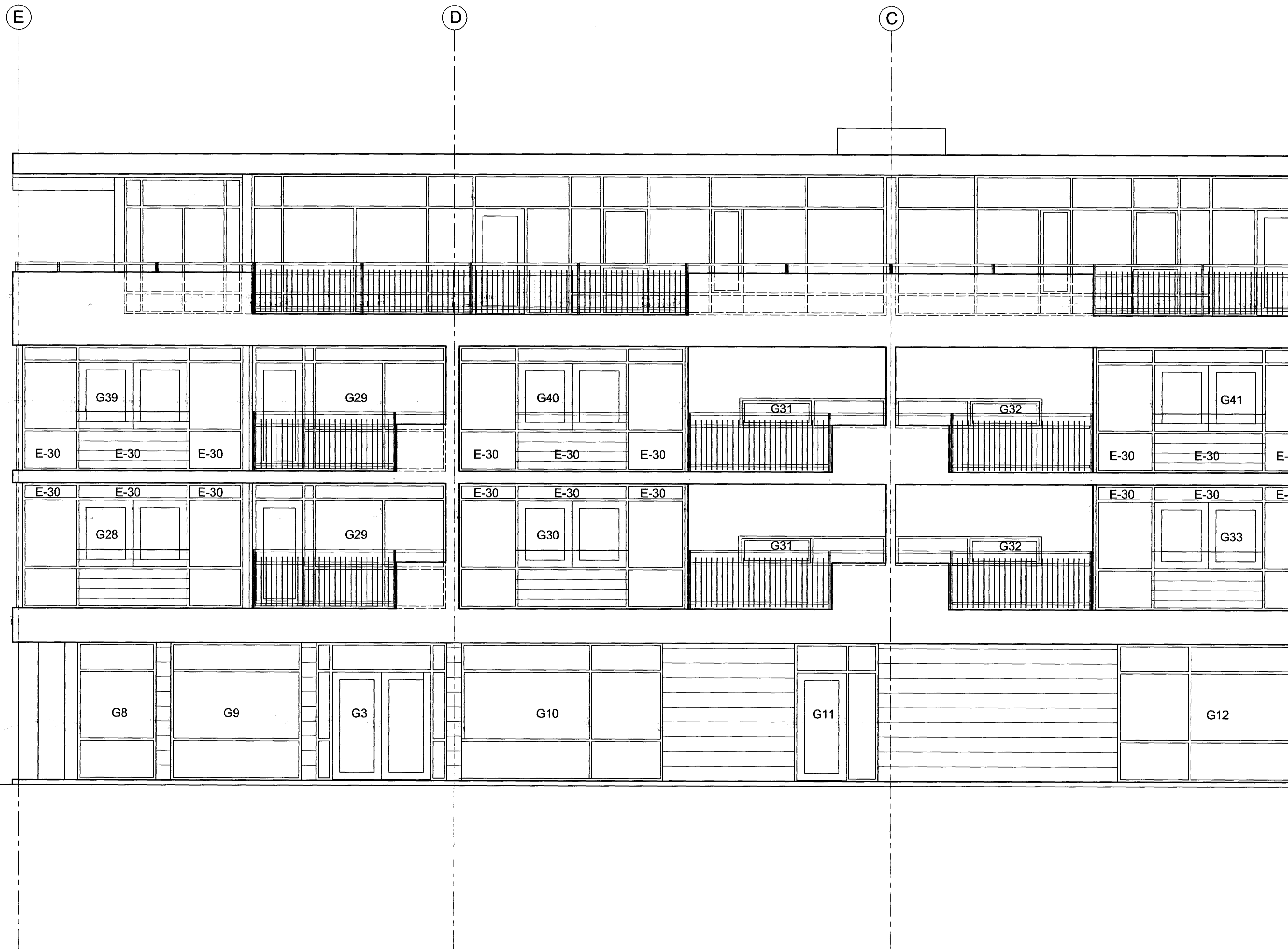
Útlit suður
