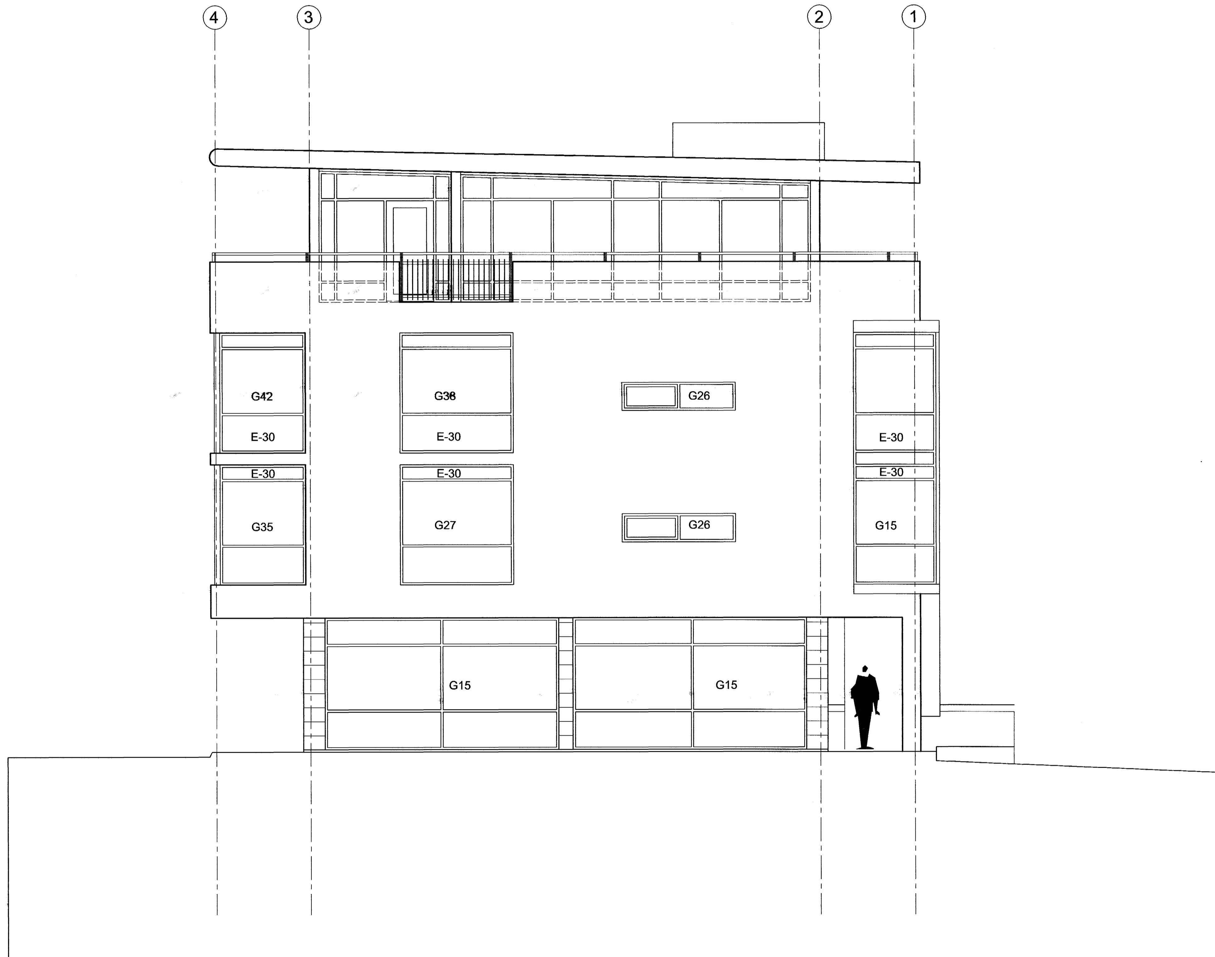
Útlit austur
