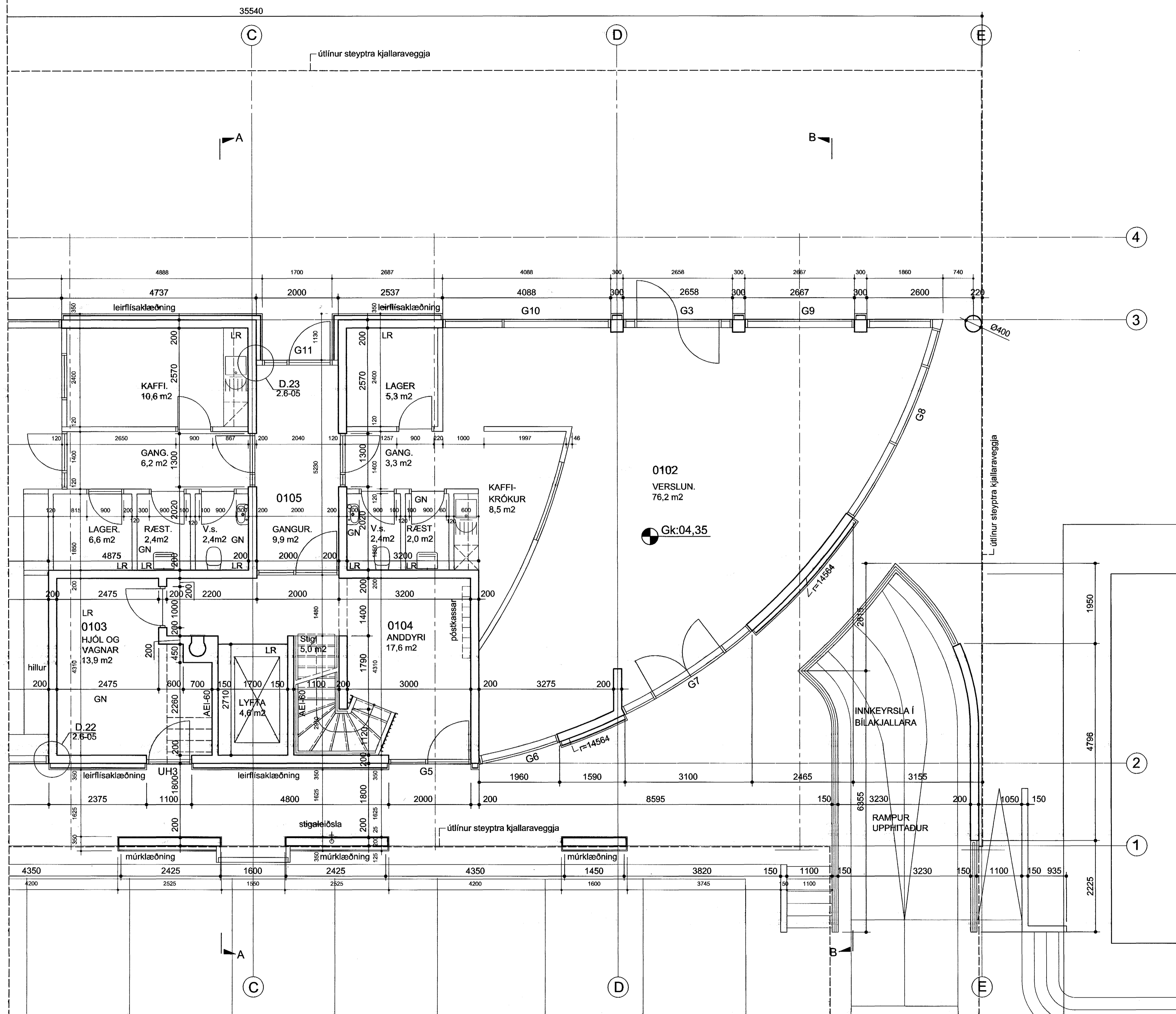
Grunnmynd 1.hæðar
