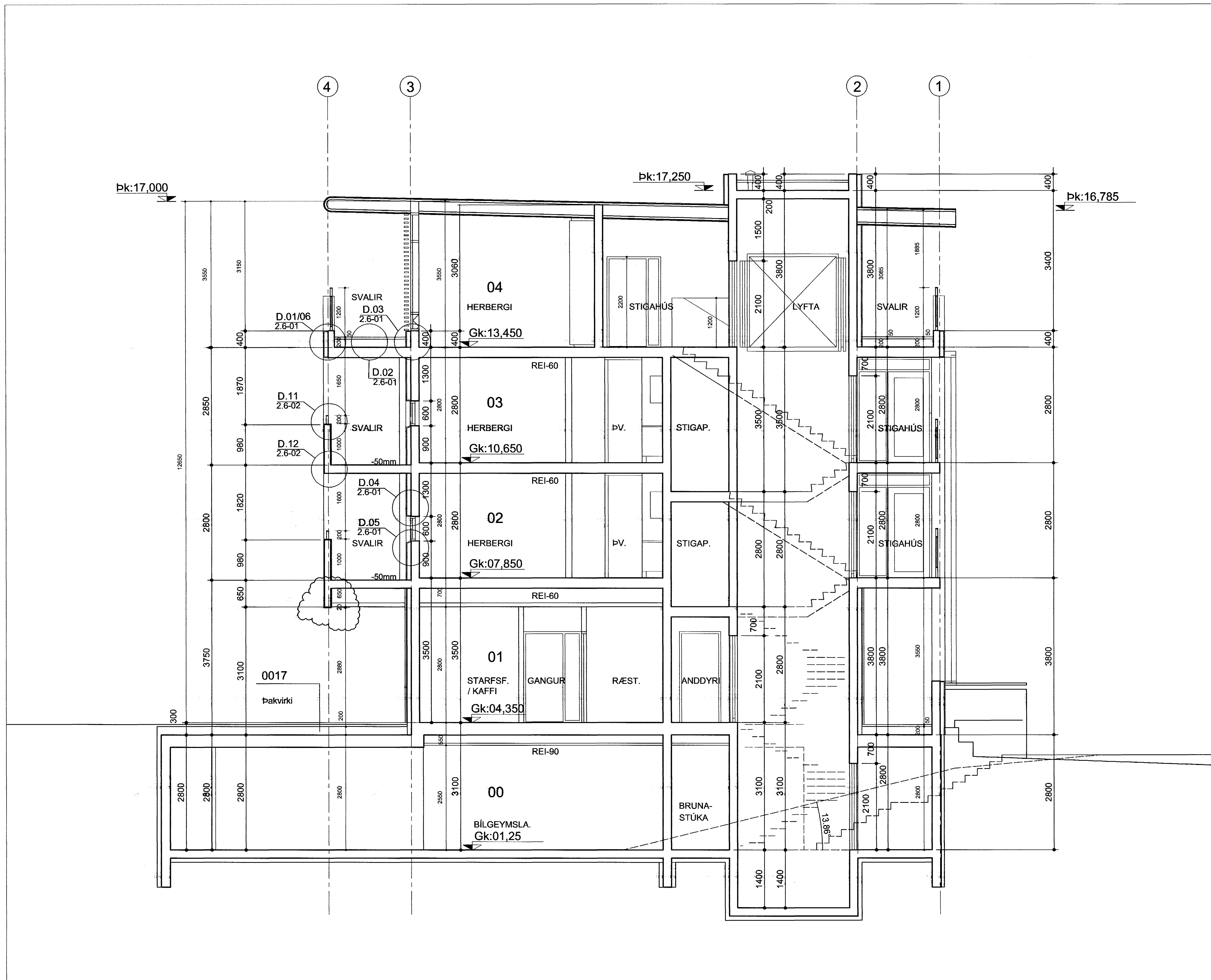
SNEIÐING A-A MKV 1:50
