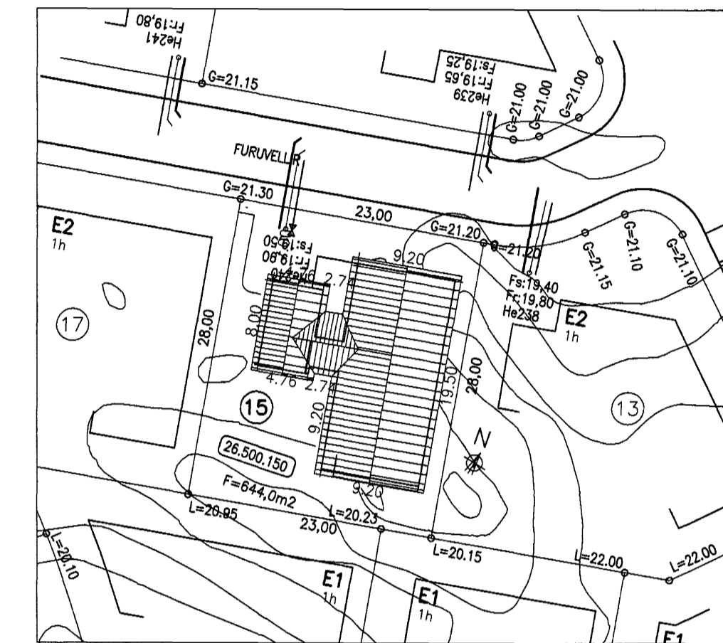
AFSTÖÐUMYND 1:500
