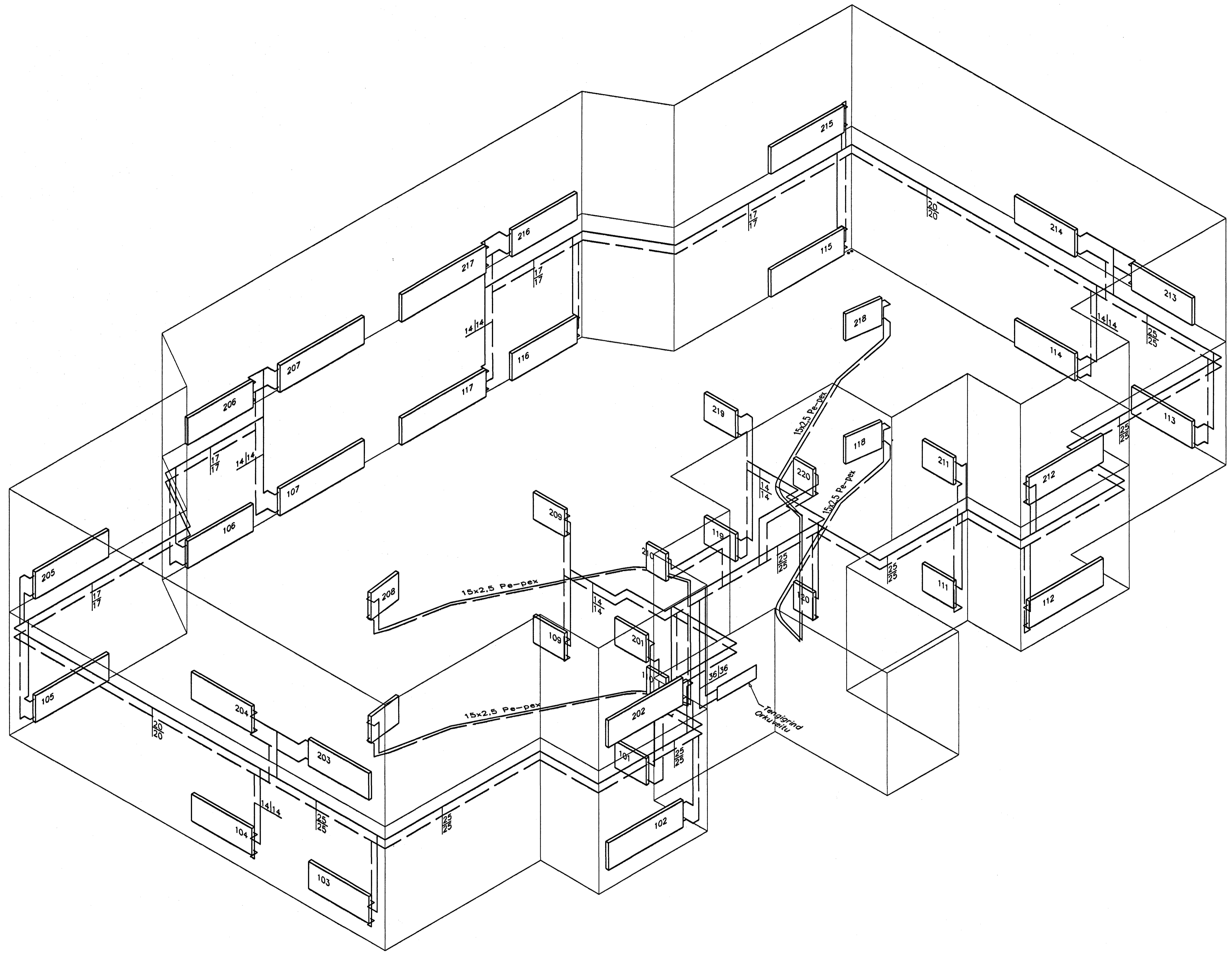
Hitalagnir, Rúmmynd, 1:50
