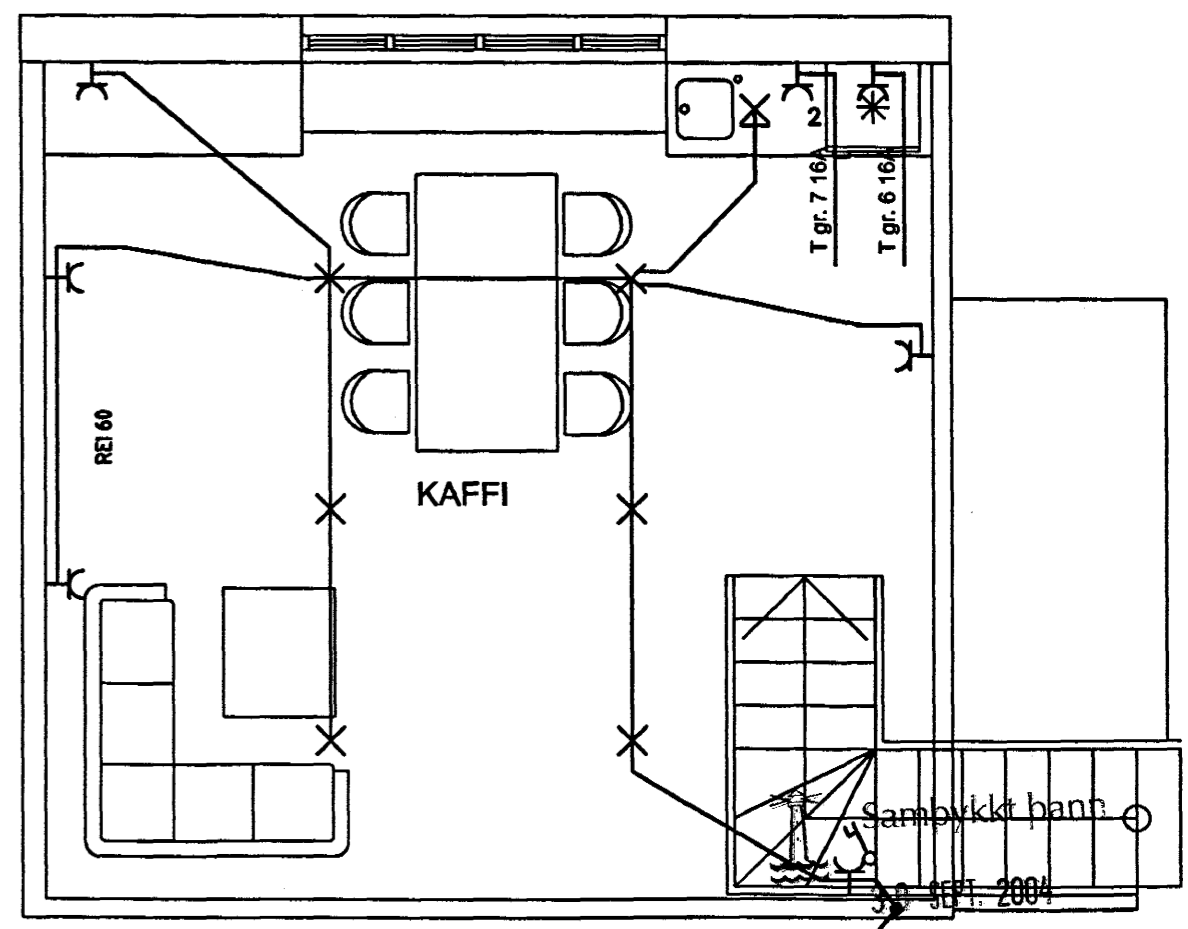
GRUNNMYND 2.HÆÐ 1:50
