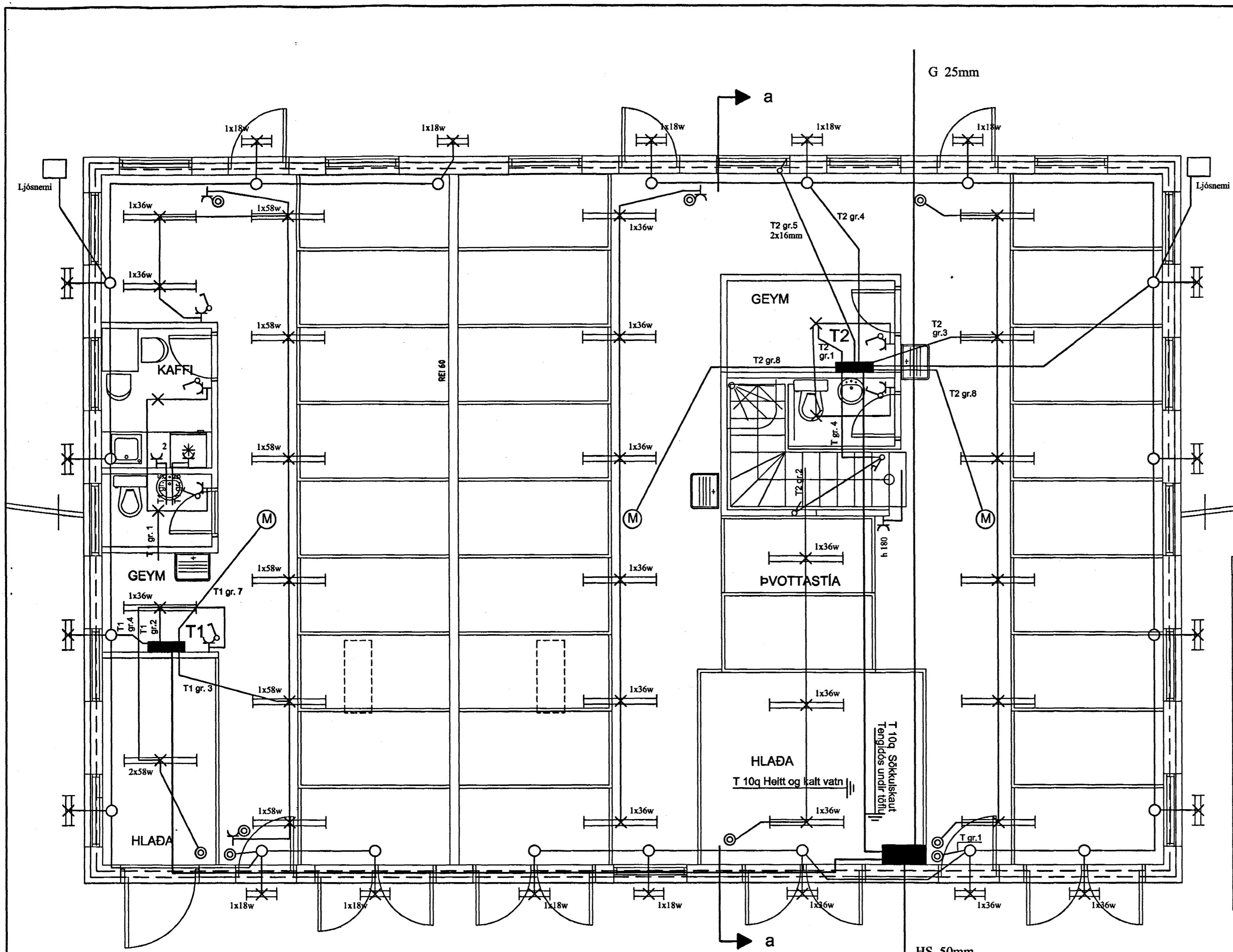
GRUNNMYND 1.HÆÐ 1:50
