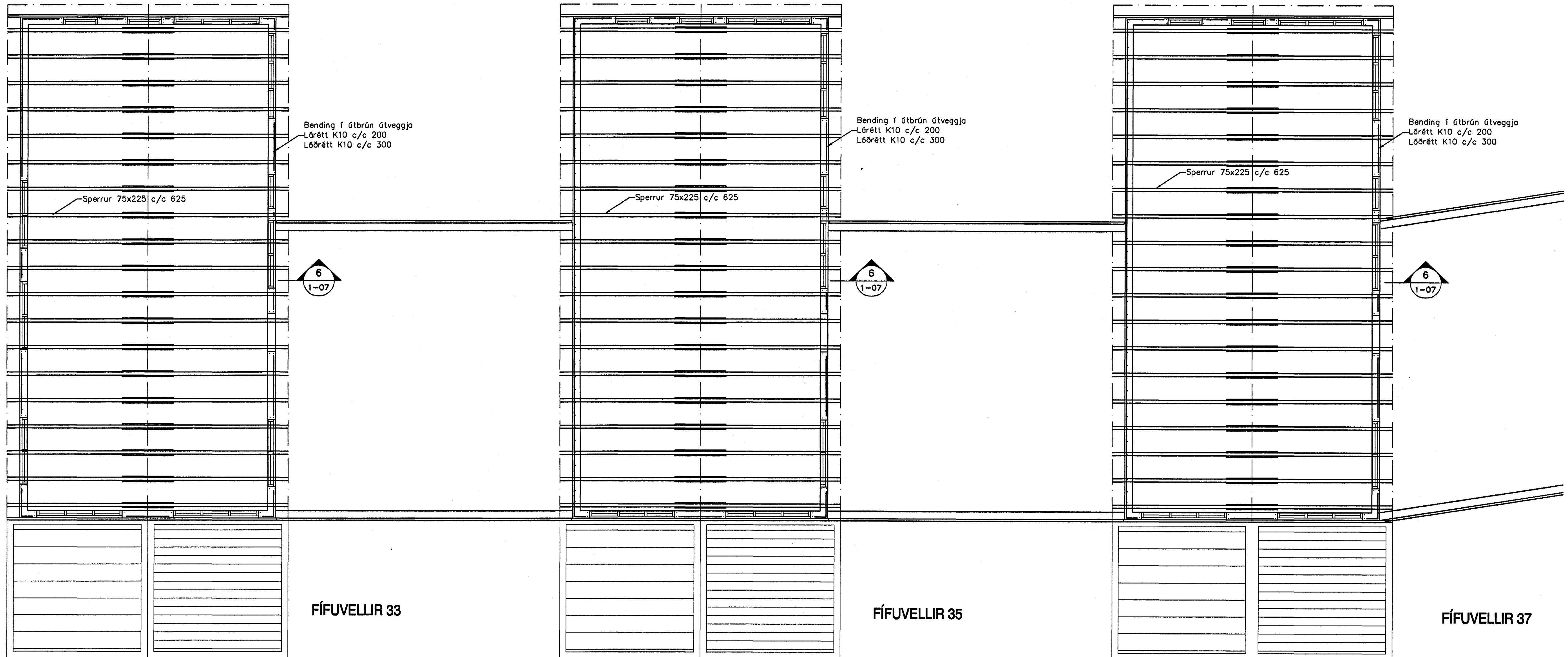
Veggir 2. hæð, þakvirki, 1:50
