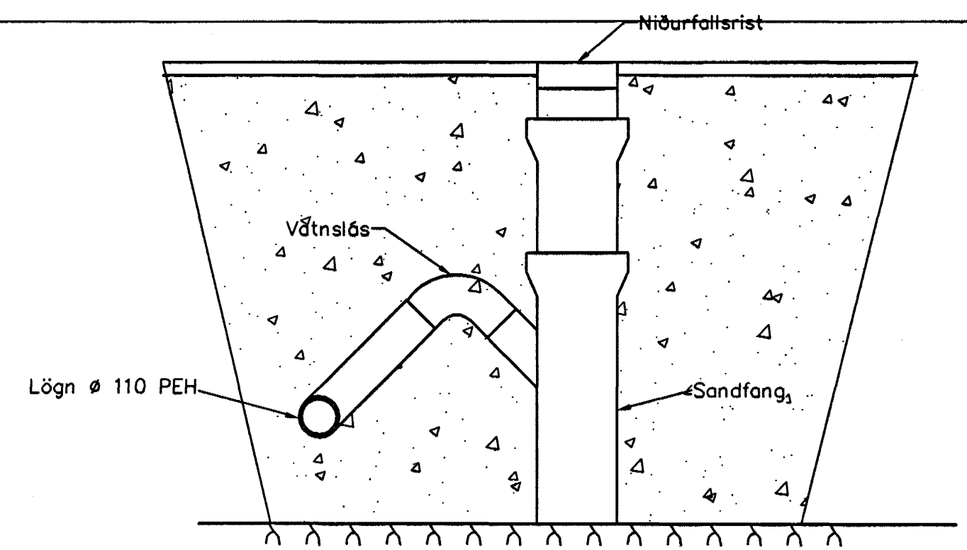
Niðurfall í plani 1:20
