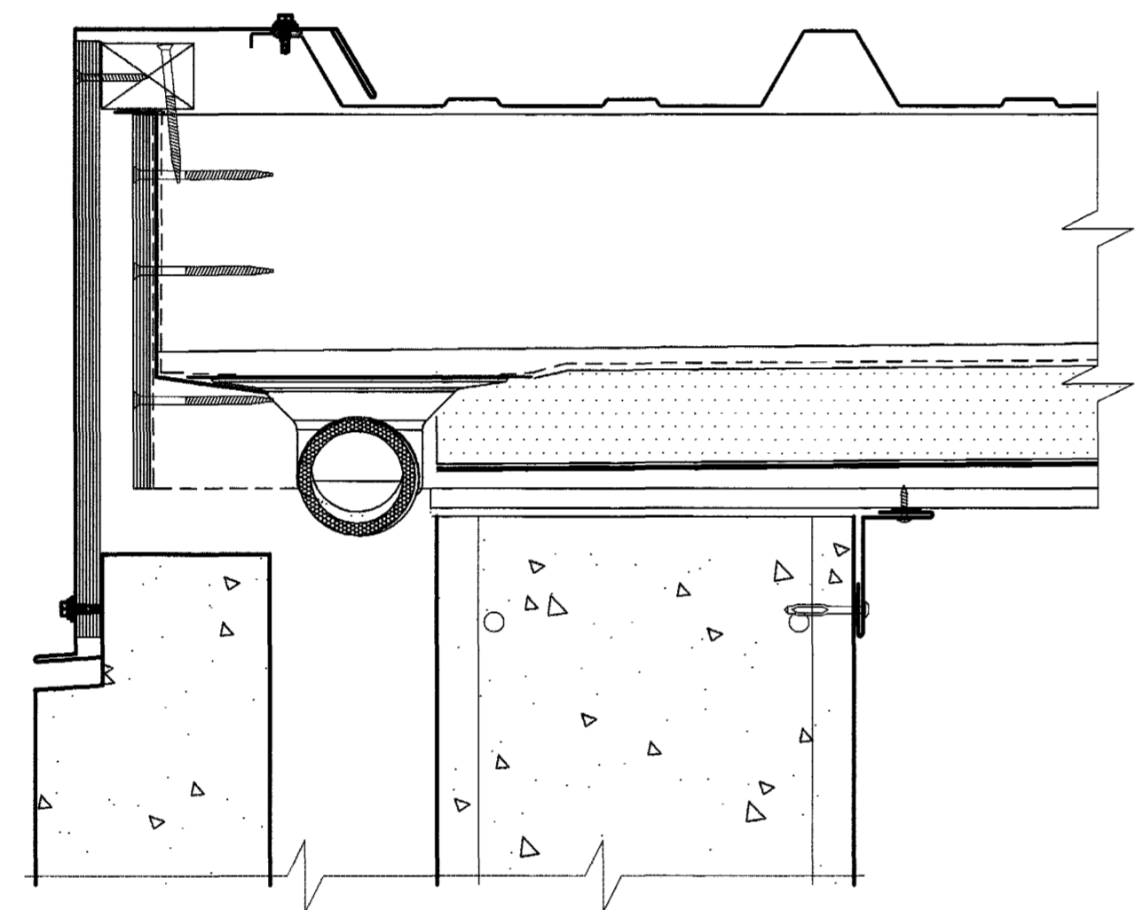
SNID A-A
