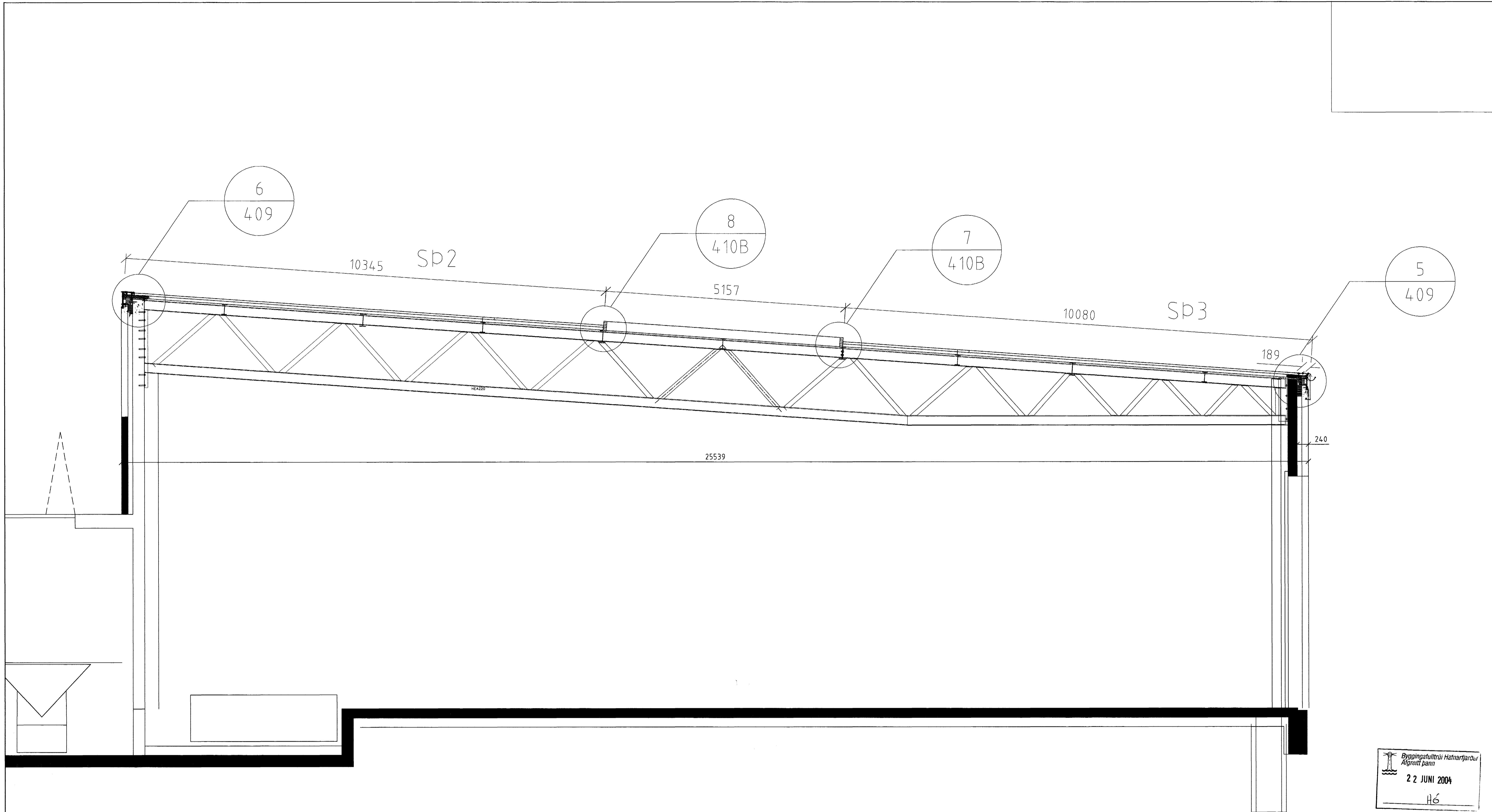
SNIÐ D-D 401
