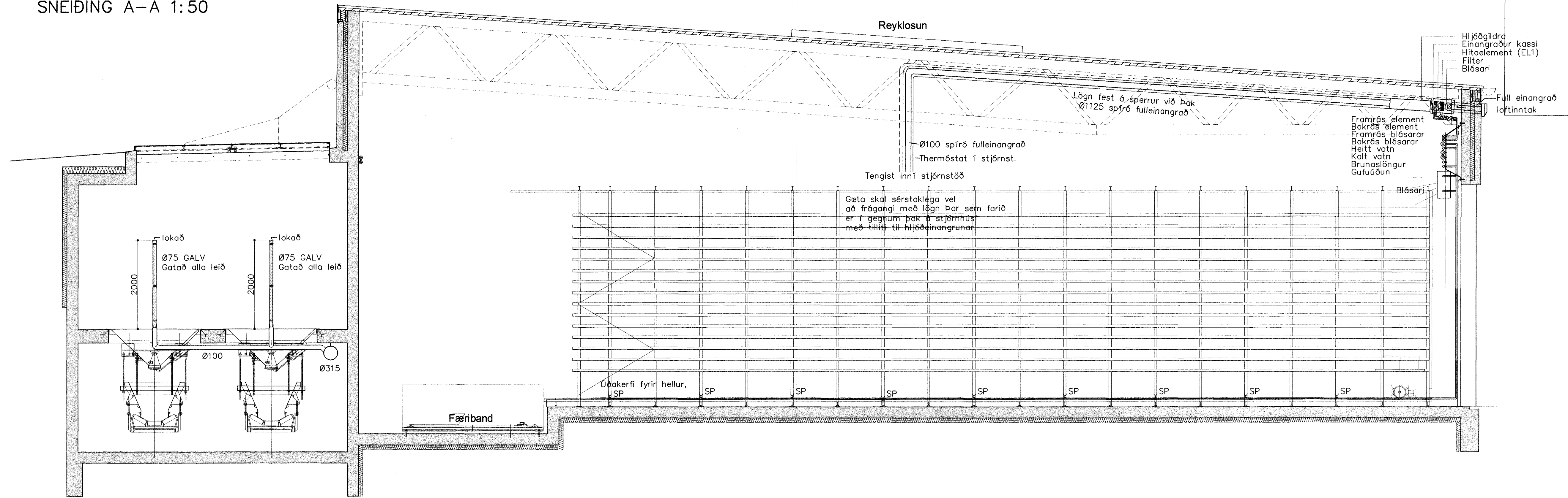
SNEIÐING A-A
