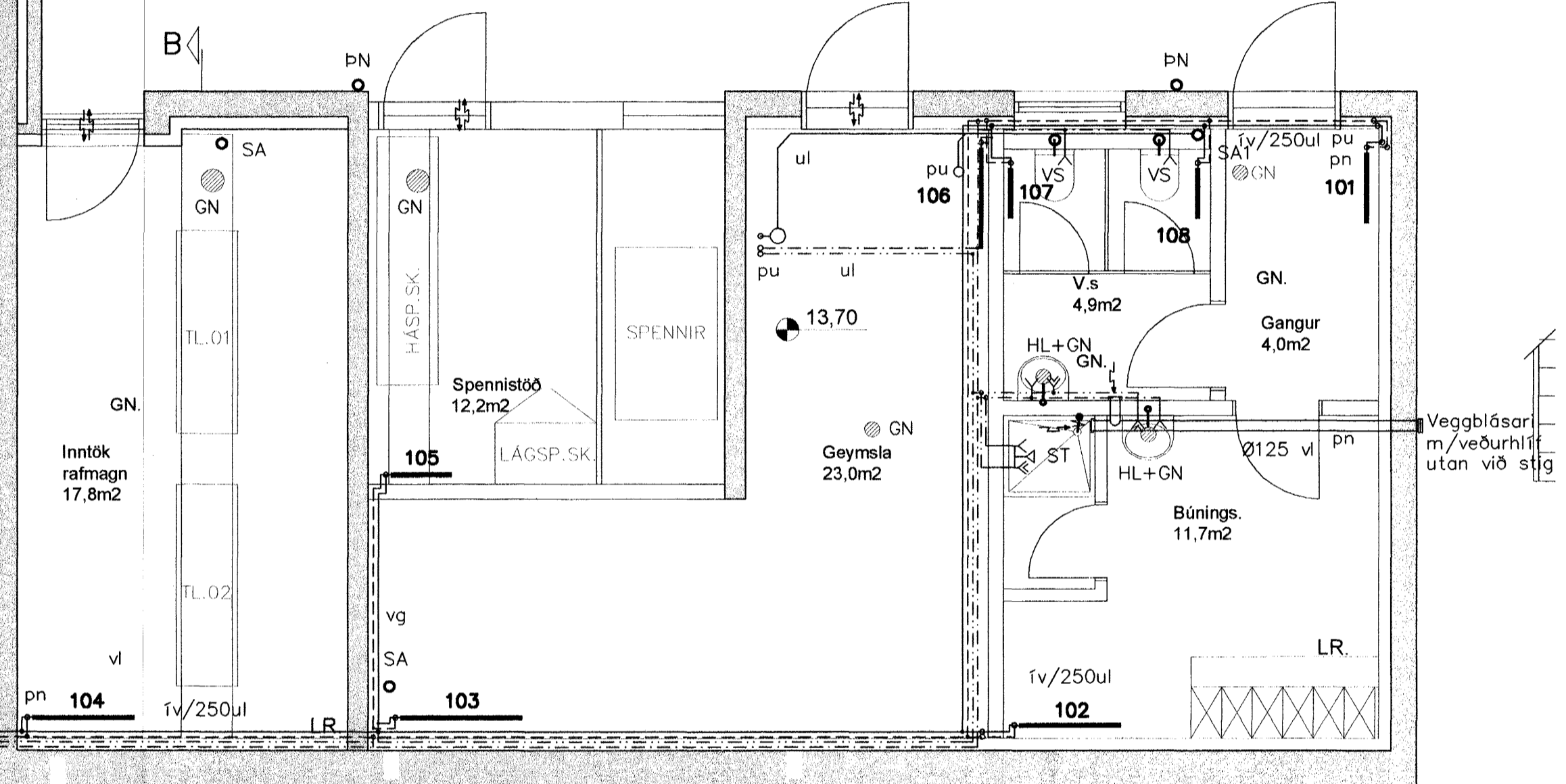
GRUNNMYND 1. hæð 1:50
