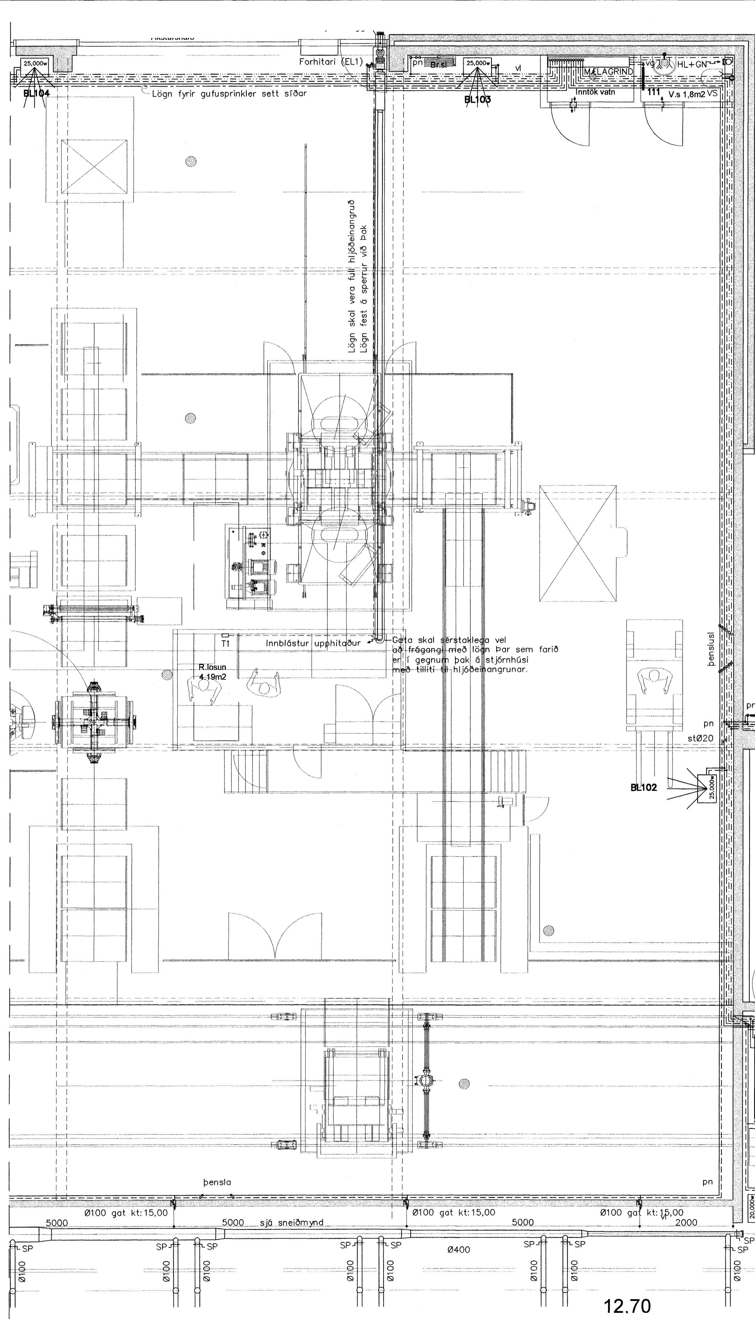
GRUNNMYND 1. hæð 1:50
