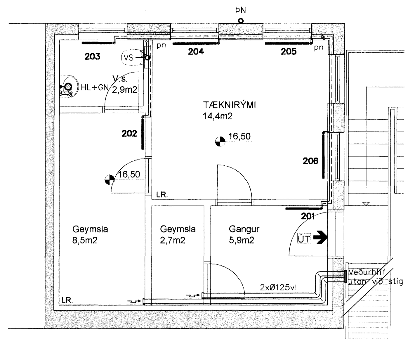
GRUNNMYND 2. hæð 1:50
