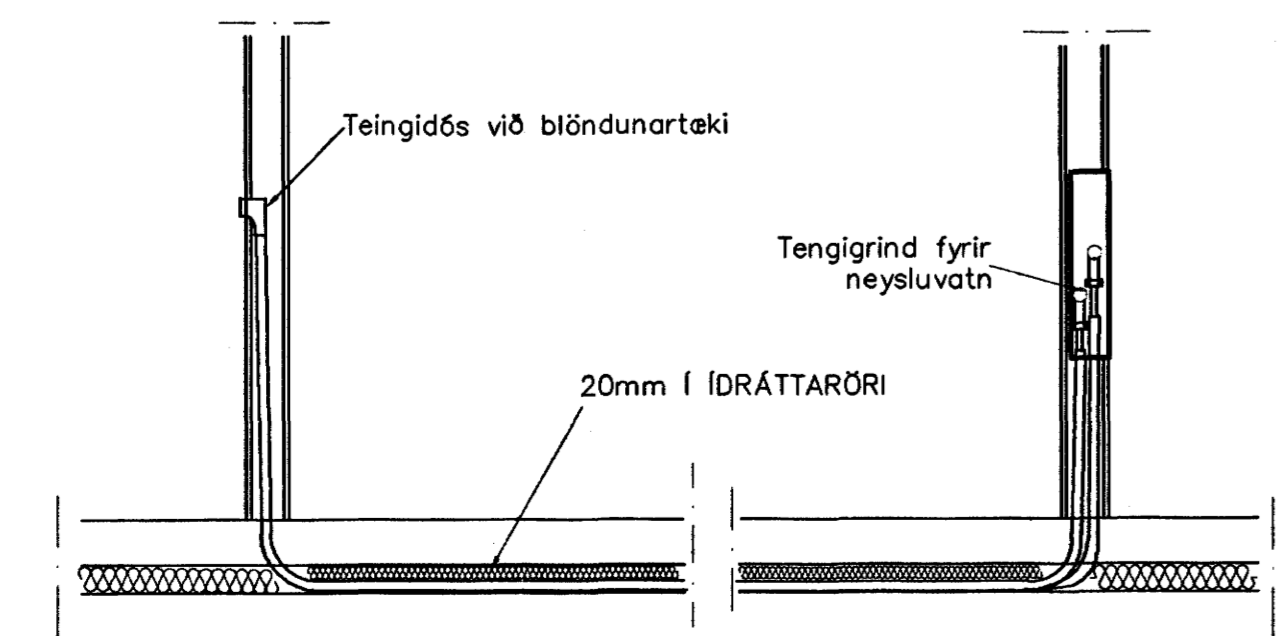
TENGING NEYSLUVATNSLAGNA 1:20
