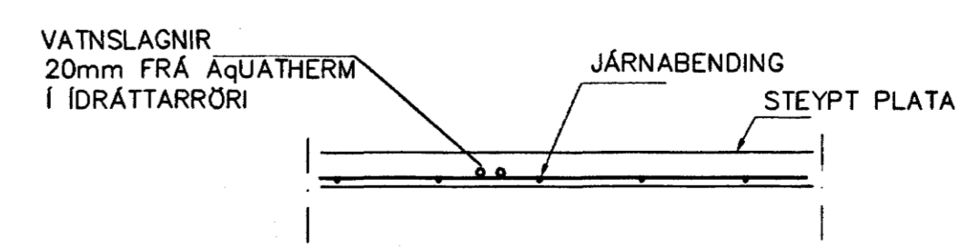
LAGNIR, SNÍÐ, 1:20
