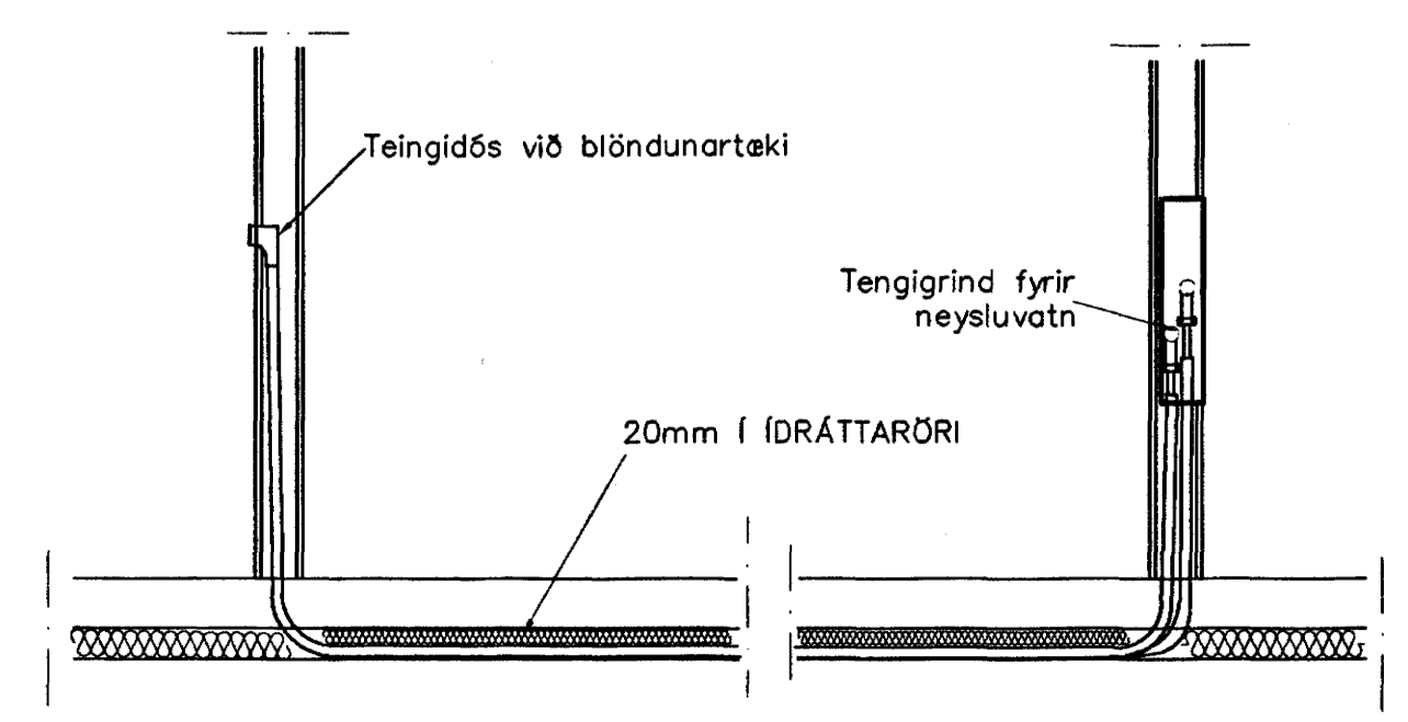
TENGING NEYSLUVATNSLAGNA 1:20
