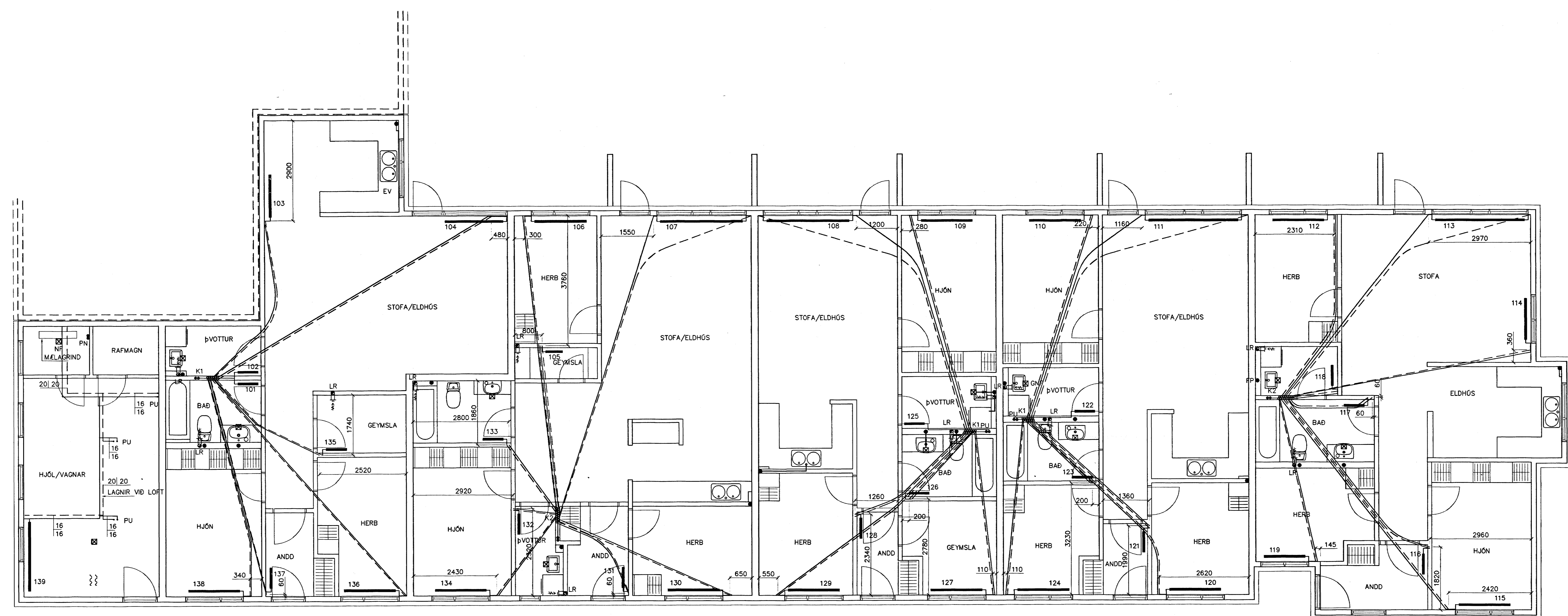
GRUNNMÝND 1 HÆÐAR 1:50
