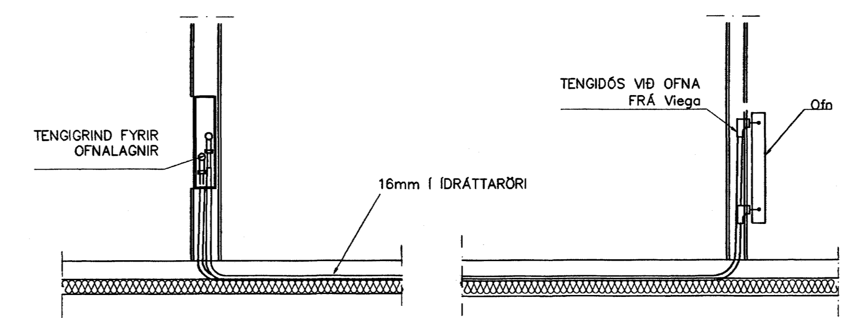
TENGING OFNALAGNALAGNA 1:20
