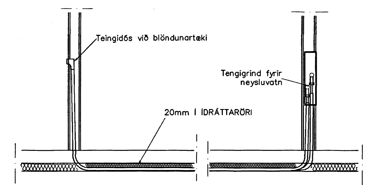
TENGING NEYSLUVATNSLAGNA 1:20
