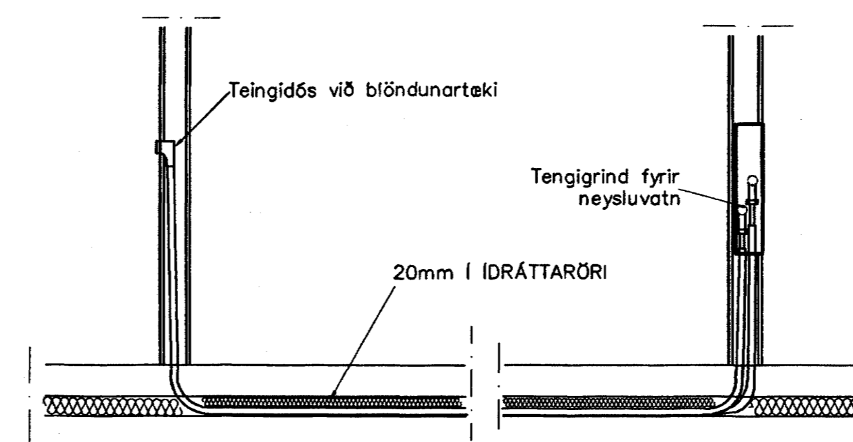
TENGING NEYSLUVATNSLAGNA 1:20
