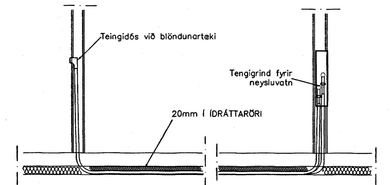
TENGING NEYSLUVATNSLAGNA 1:20
