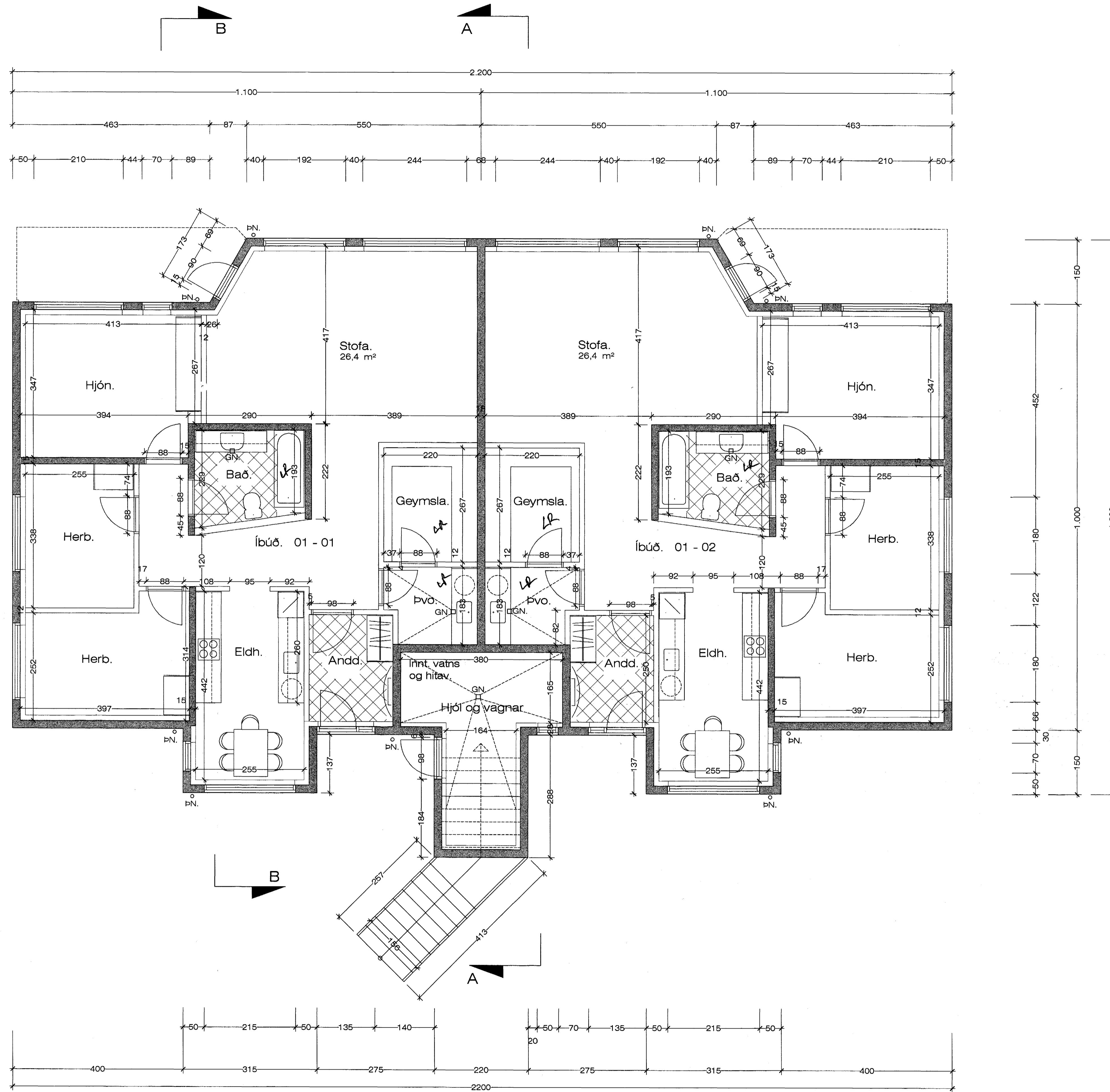
Grunnmynd 1. Hæð. 1:50
