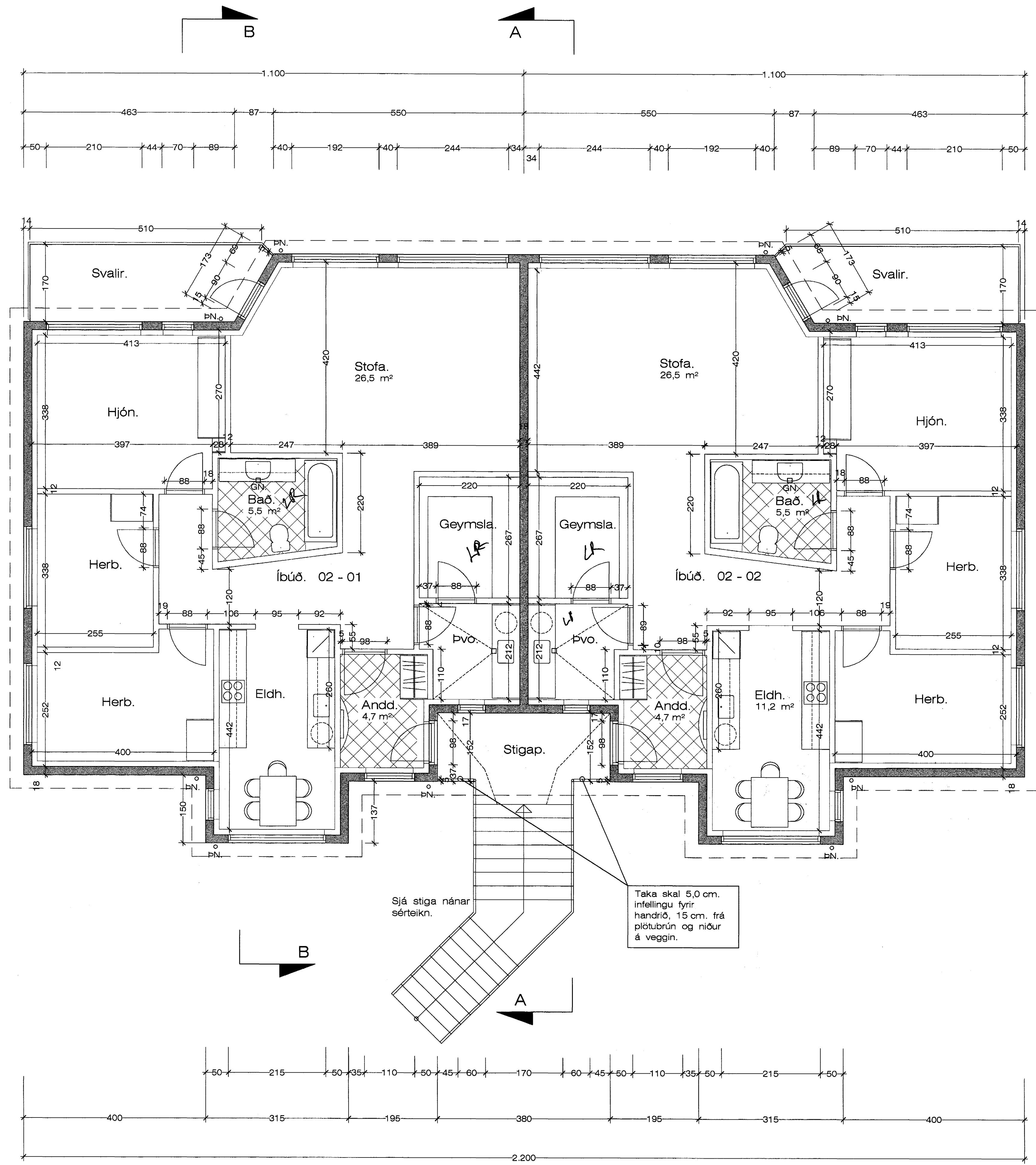
Grunnmynd. 2. Hæð. 1:50
