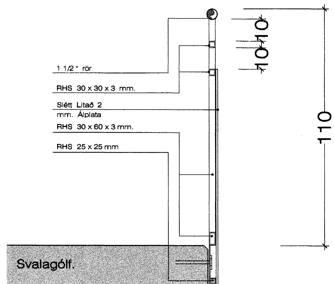
Svalahandrið. 1:10
