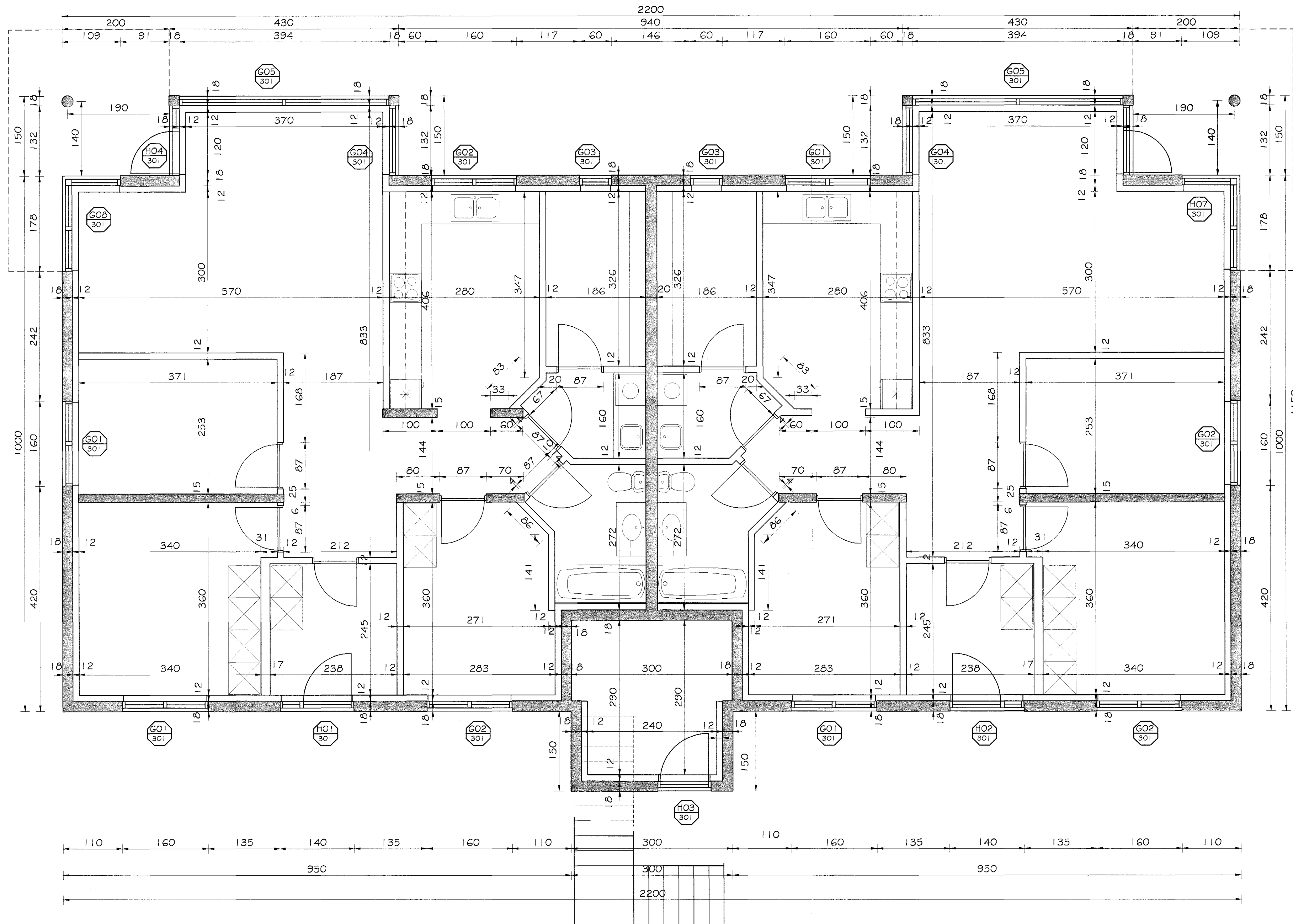
GRUNNMYND NEDRI HÆÐAR MKV. 1:50
