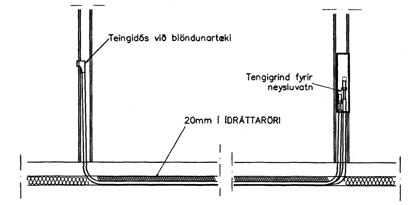
TENING NEYSLUVATNSLAGNA 1:20
