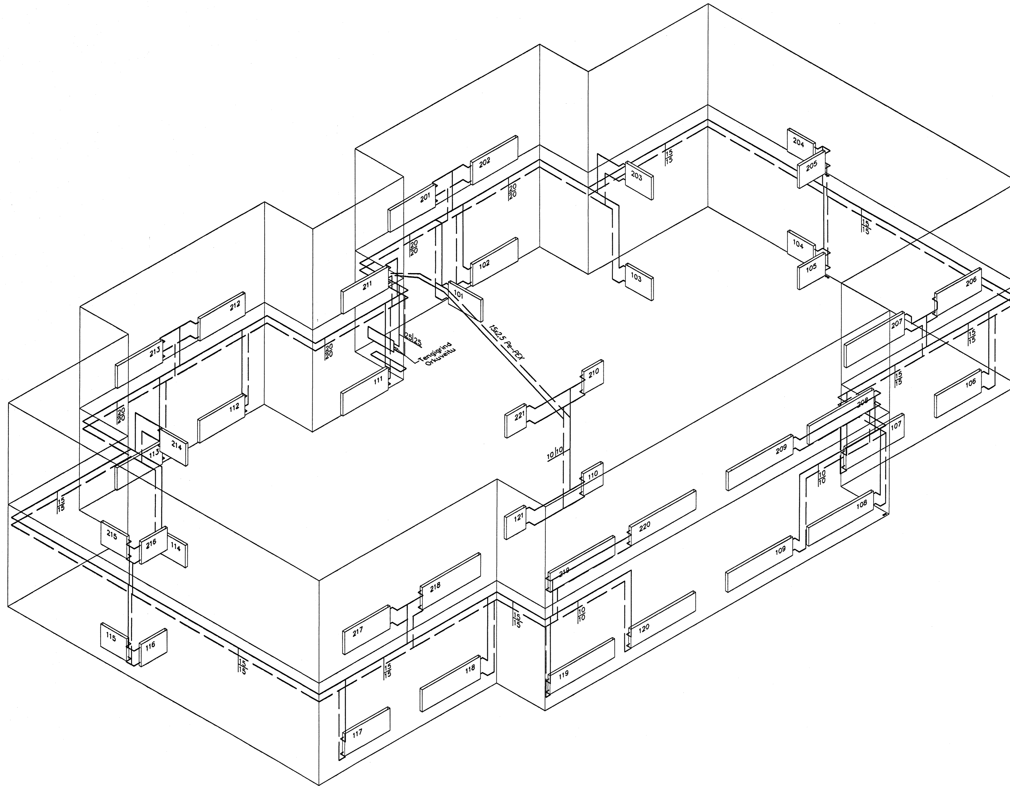
Hitlag, Rúmmynd, 1:50
