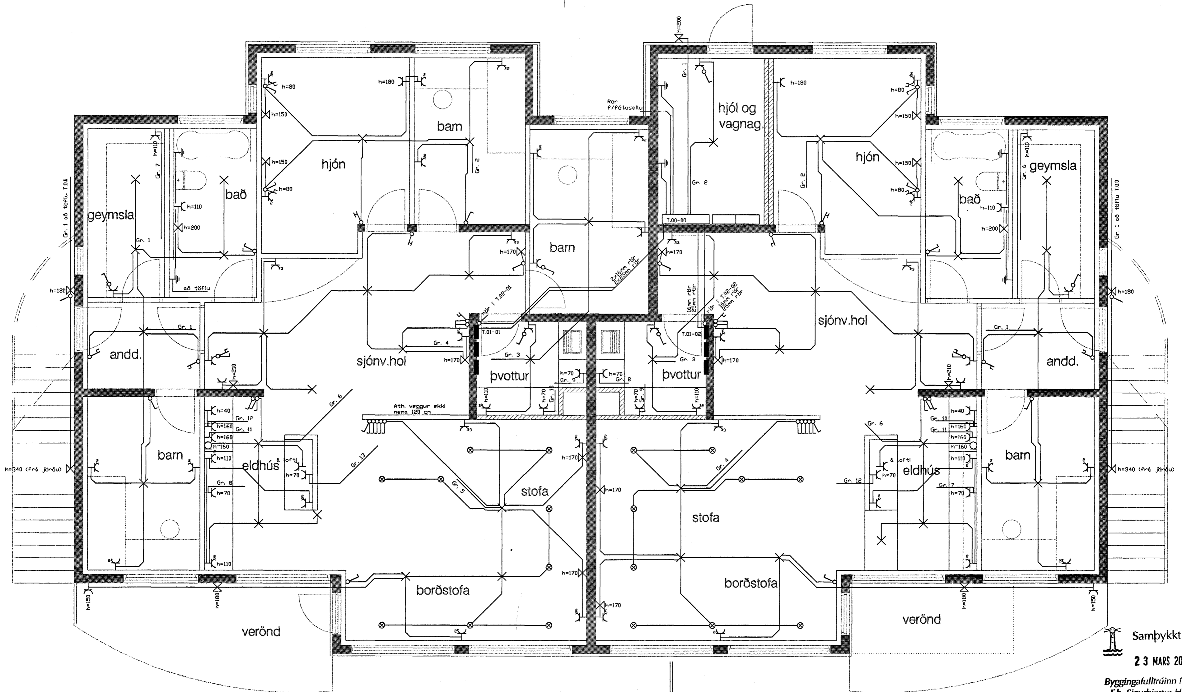
grunnmynd 1. hæð
