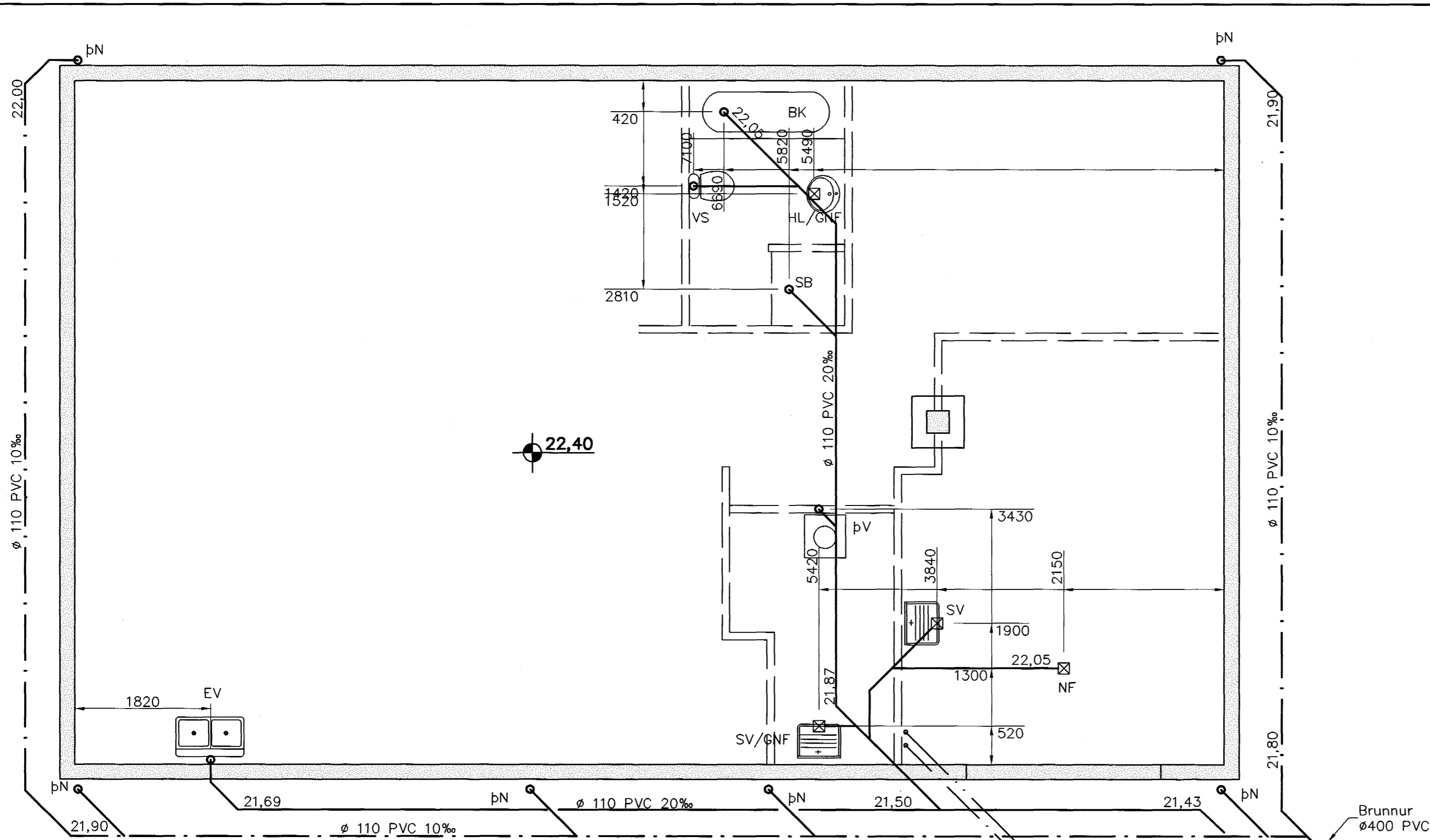
Grunnlagnir, Grunnmynd, 1:50
