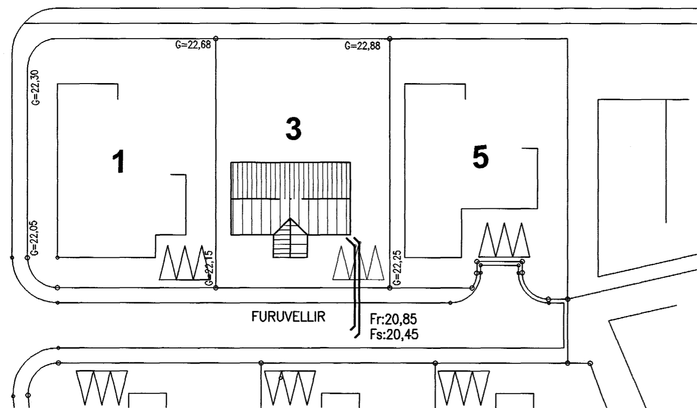
Afstöðumynd, 1:500
