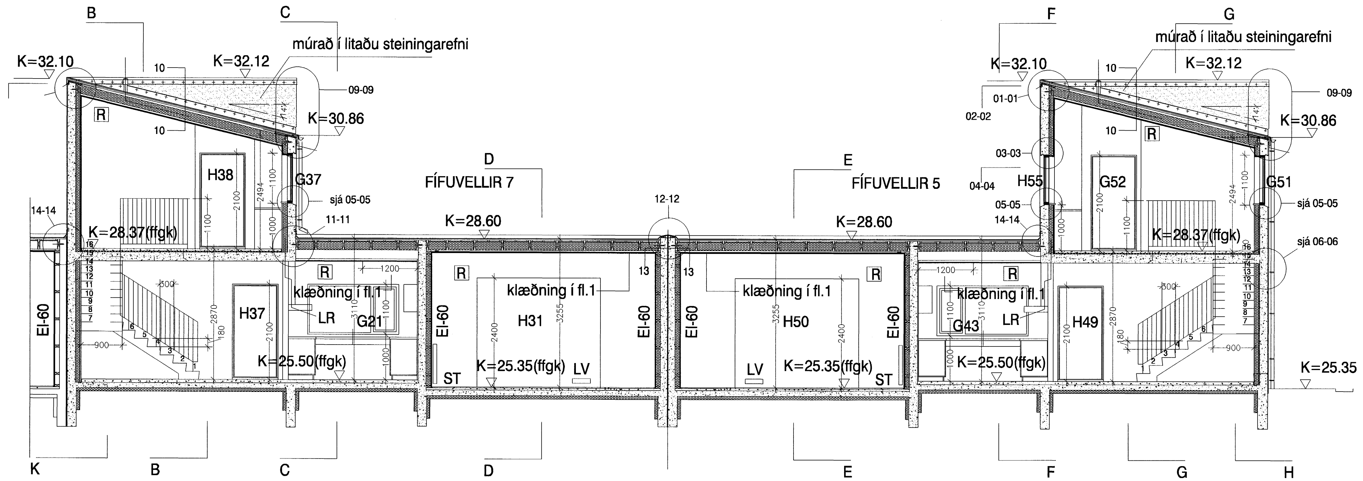
SNEIÐING A - A FÍFUVELLIR 7 OG FÍFUVELLIR 5 MKV: 1:50 ATH: ALLAR SNEIÐMYNDINAR ER TEKINAR HORNRÉTT Á 90° GEGNUM HÚSALENGJUNA
