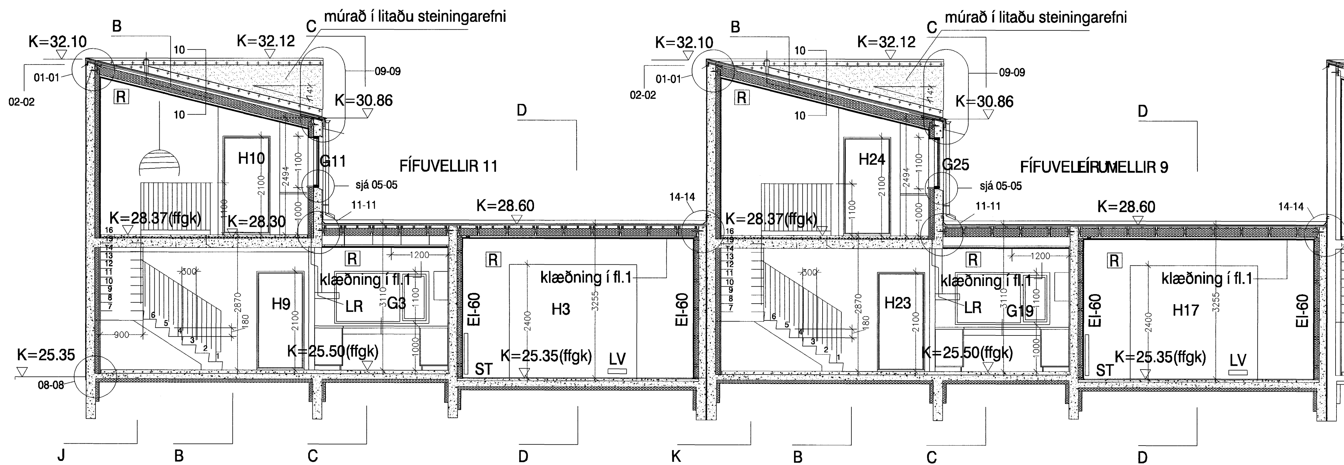
SNEIÐING A - A FÍFUVELLIR 11 OG FÍFUVELLIR 9 MKV: 1:50 ATH: ALLAR SNEIÐMYNDINAR ER TEKINAR HORNRÉTT Á 90° GEGNUM HÚSALENGJUNA
