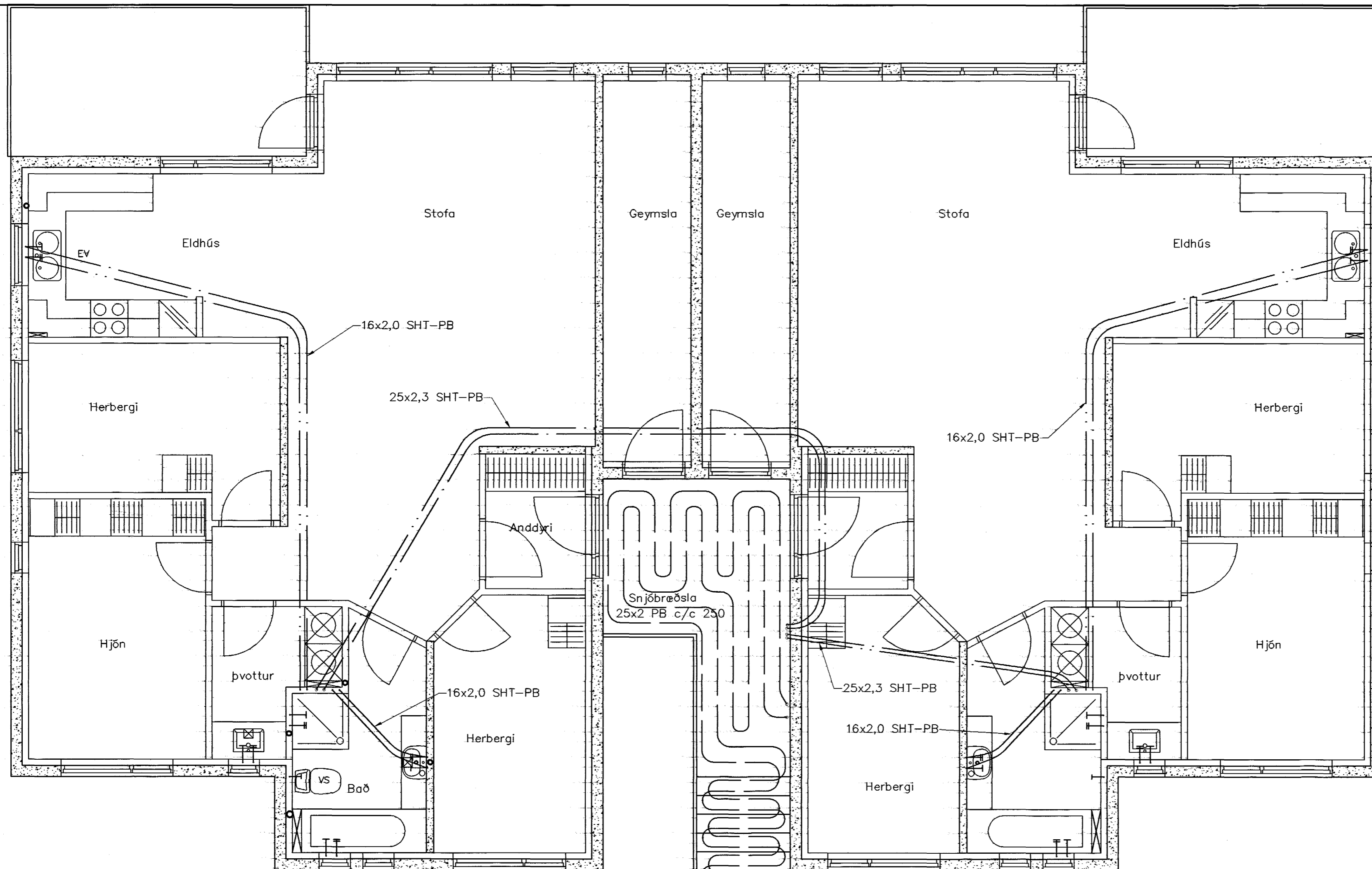
Neysluvatn Stofnlagnir 2. hæð, Grunnmynd, 1:50
