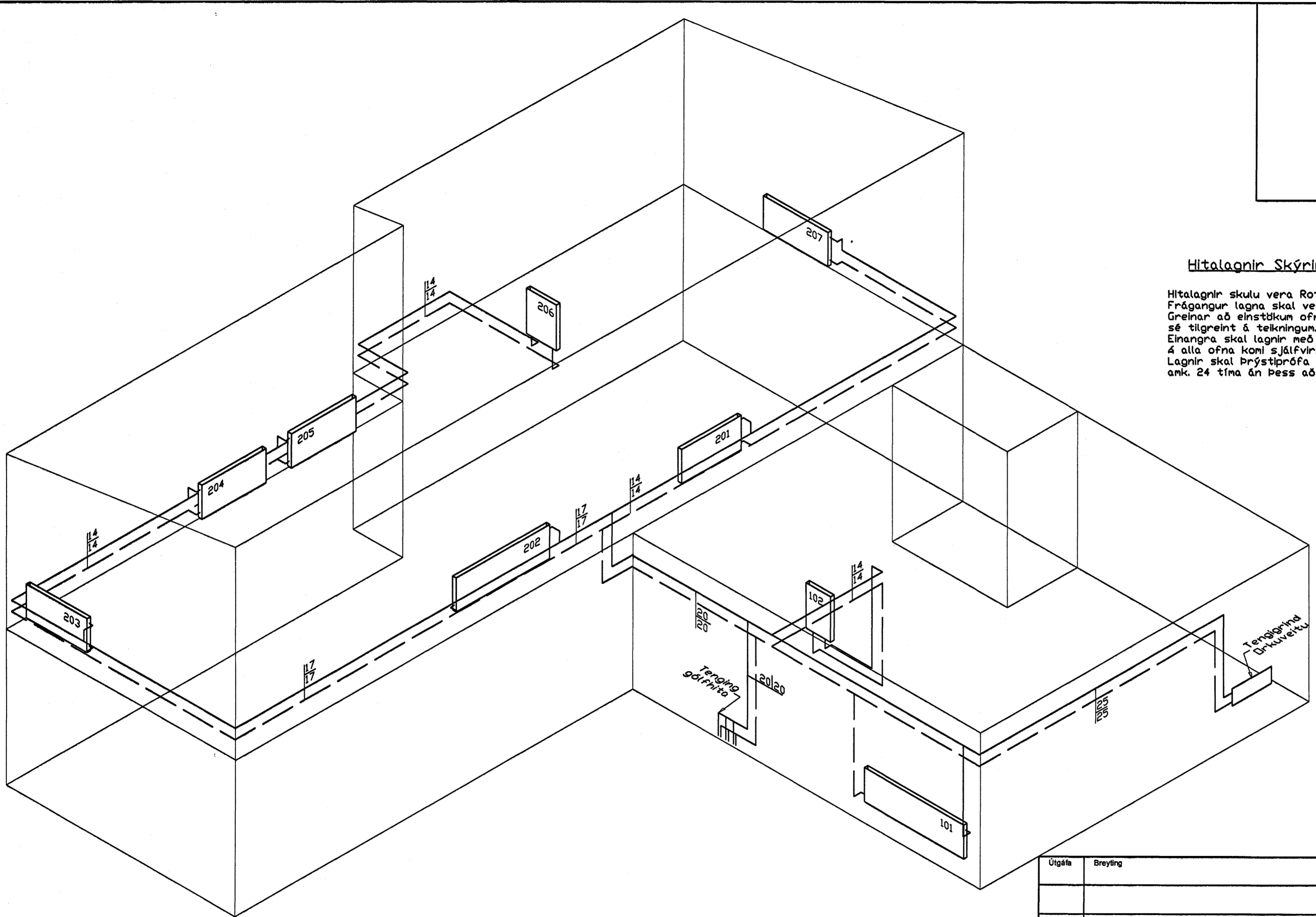
Hitalagnir, Rúmmynd, 1:50
