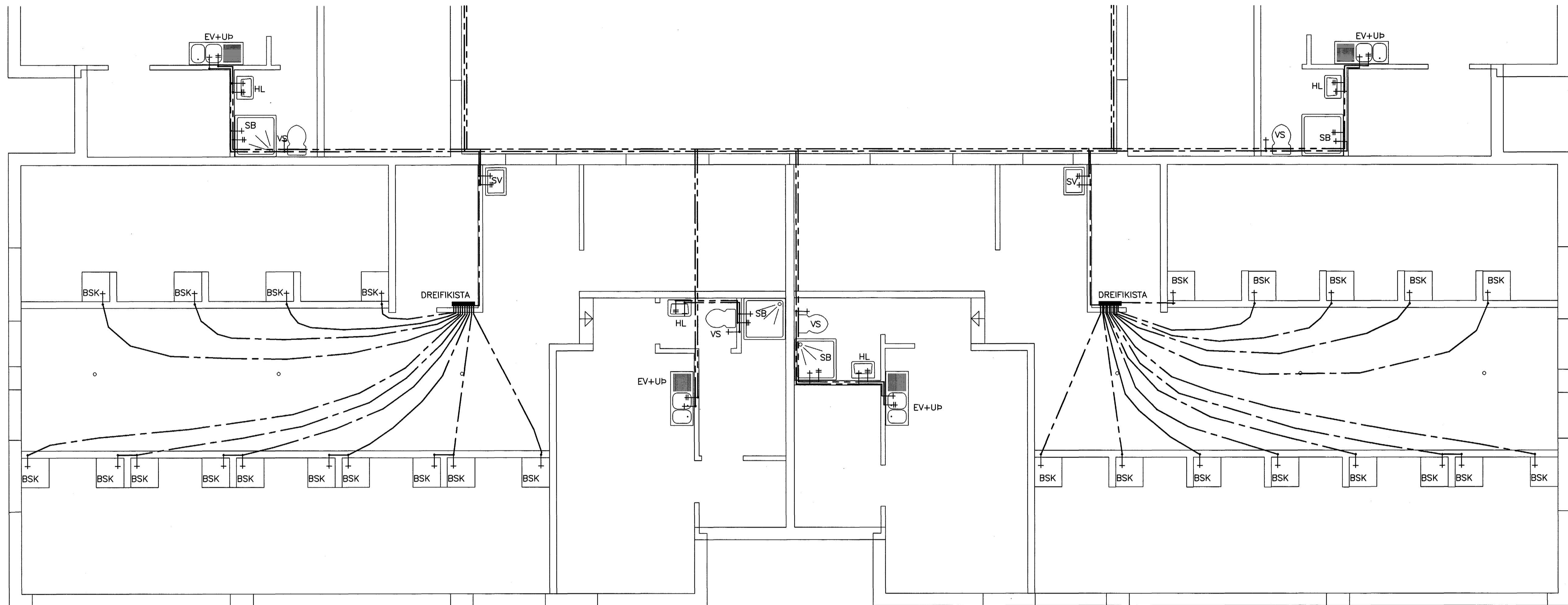
GRUNNMYND, 1:50
