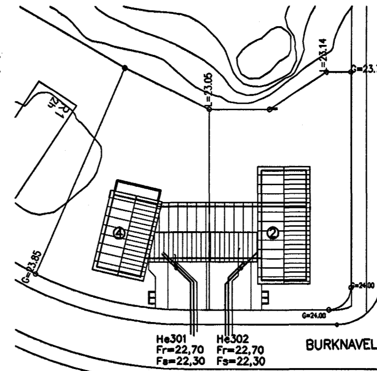
Afstöðumynd, 1:500
