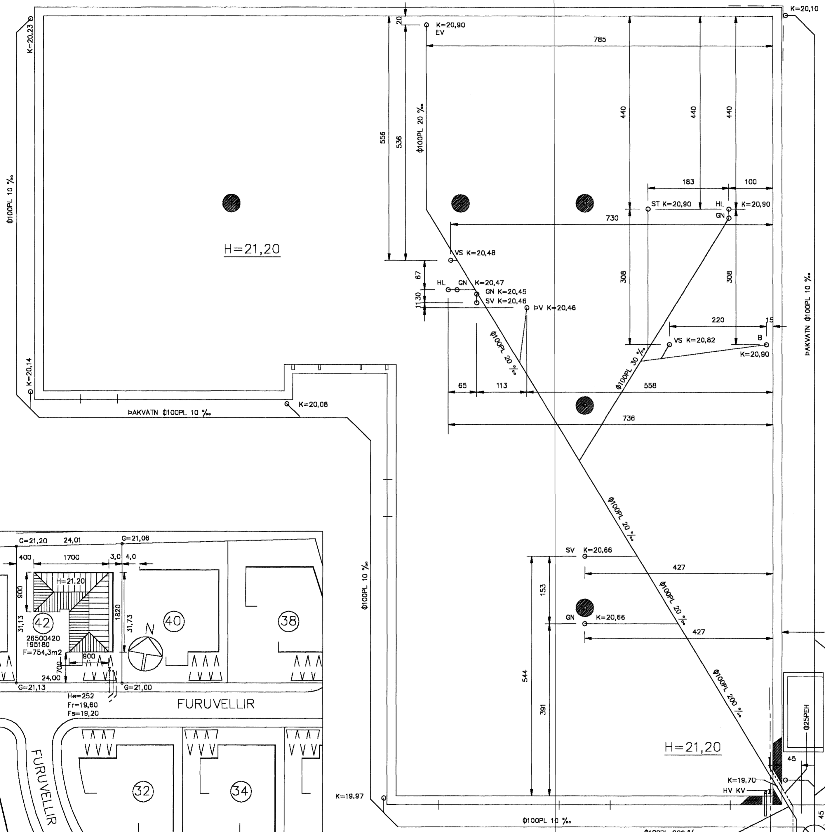
GRUNNMYND, M=1:50
