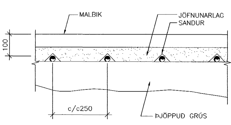
B SNID 1:10 MALBIK
