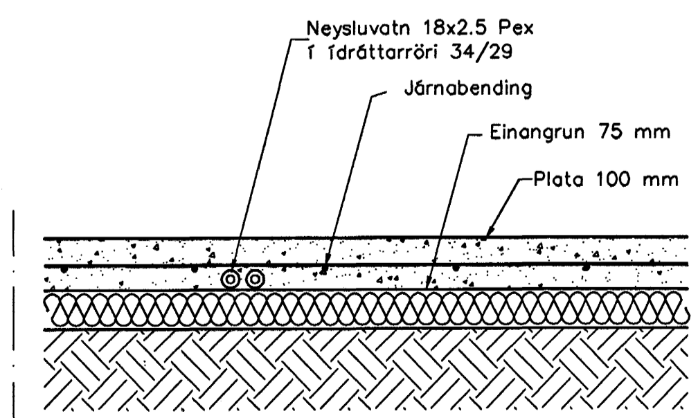
Neysluvatnslagnir, Snið í botnplötu. 1:10
