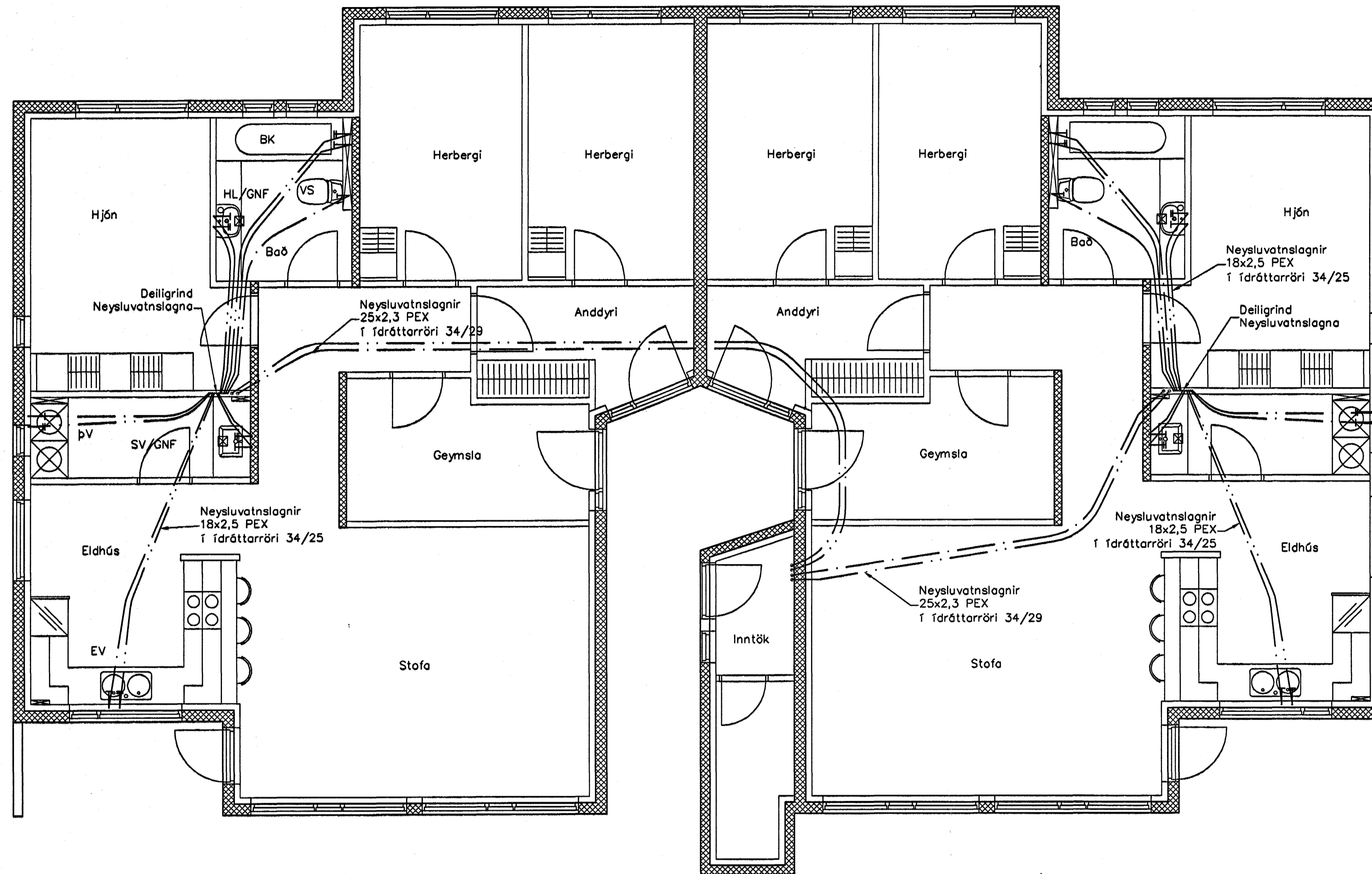
Neysluvatnslagnir 1. hæð. 1:50
