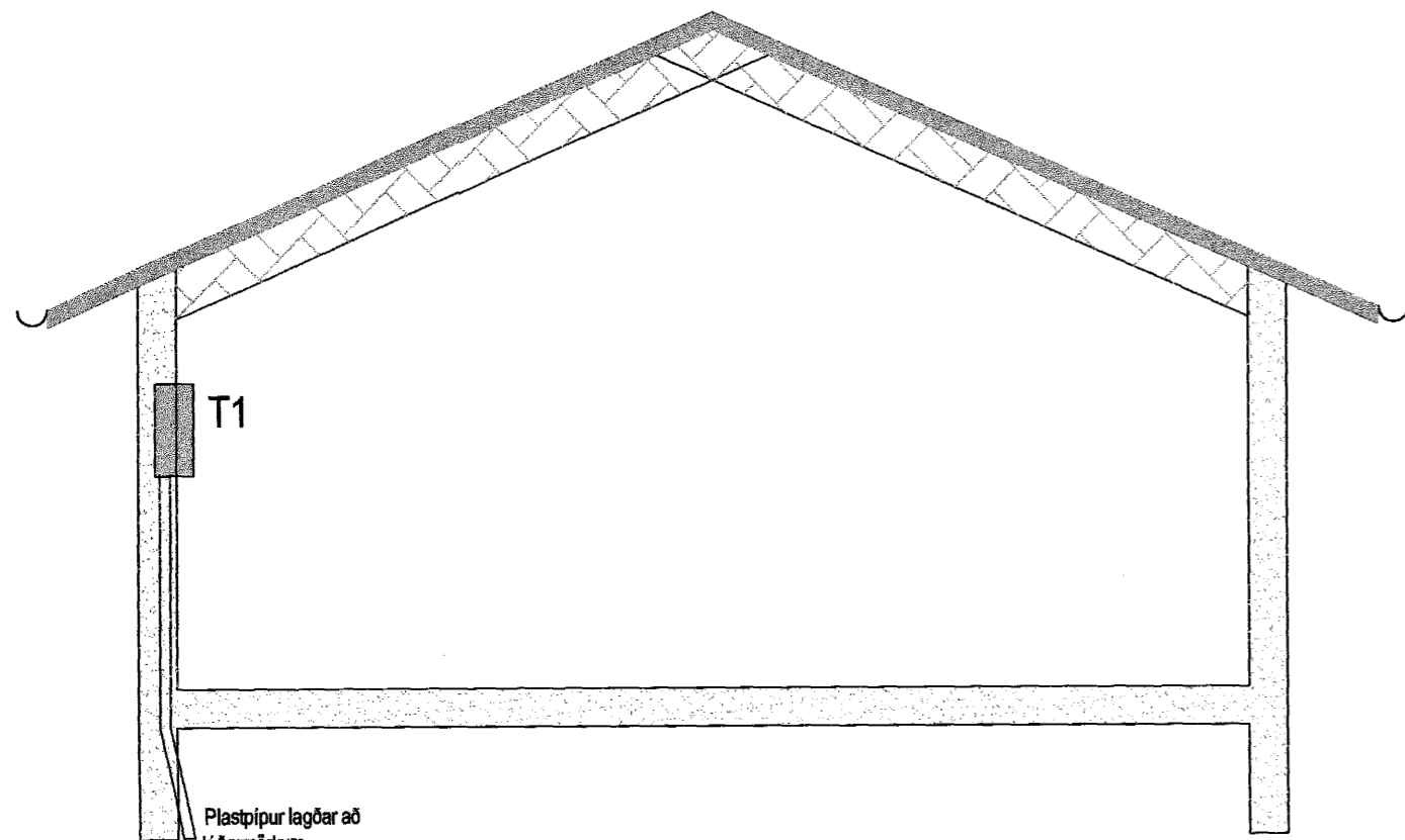
Snið A-A
