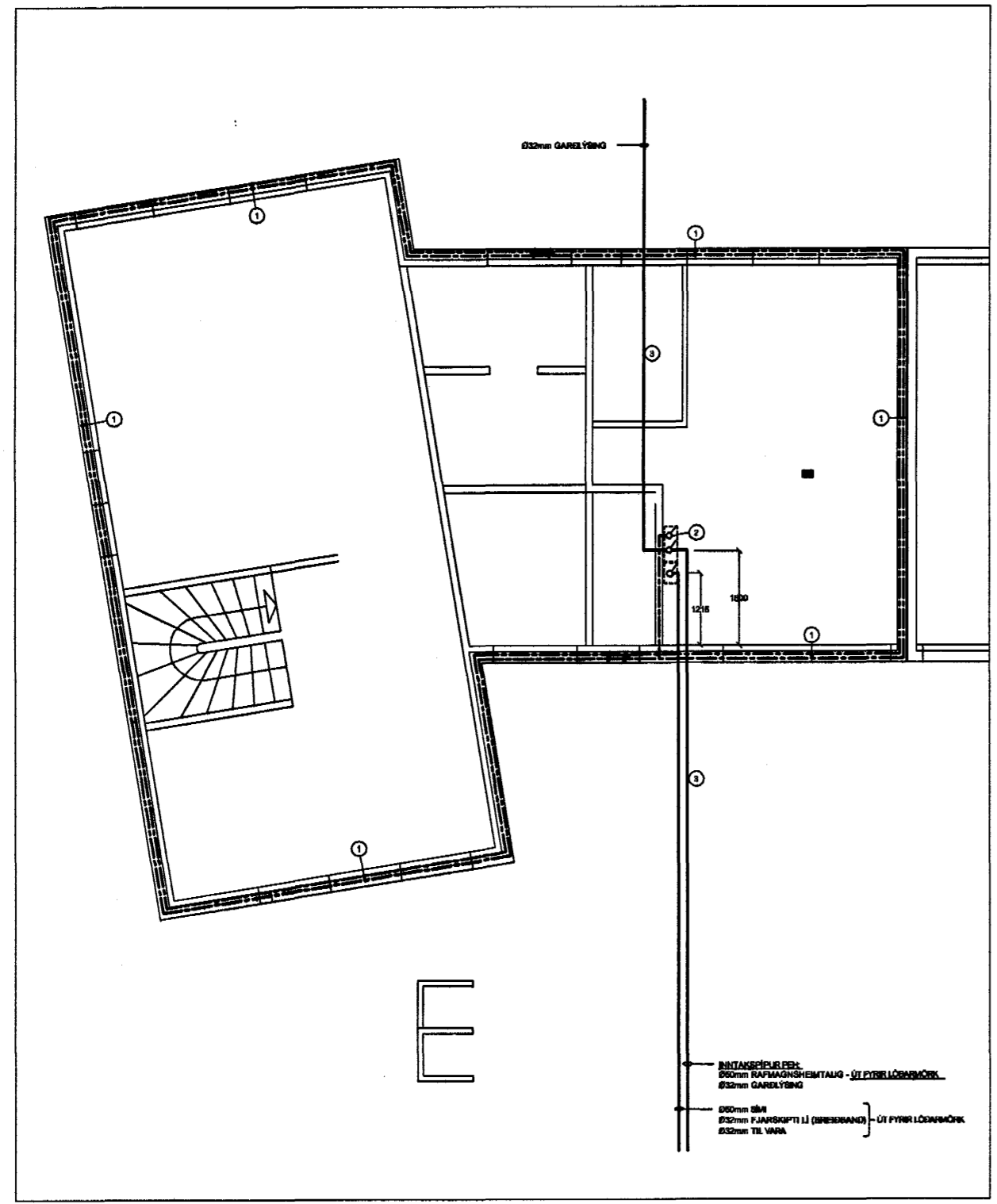
GRUNNMYND, MKV. 1:100
