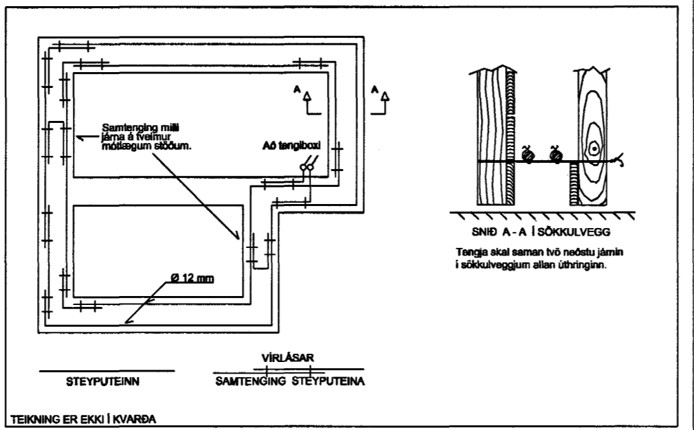
FYRIRMYND GRUNNMYND SÖKKULVEGGJA DÆMIGERÐUR FRÁGANGUR
