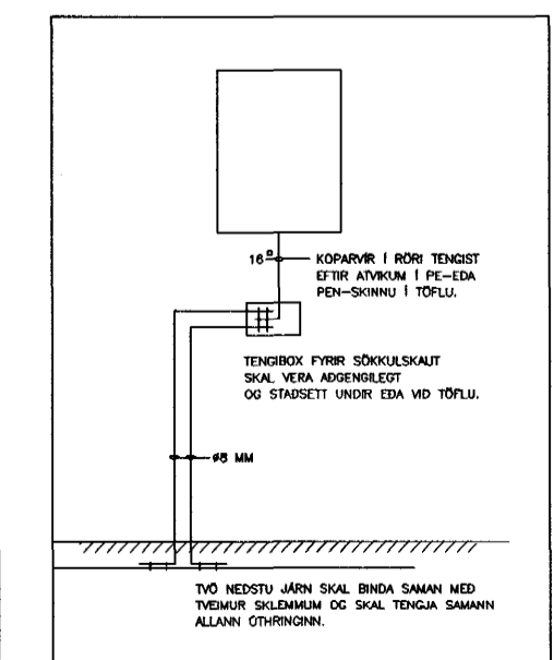
SNID FRÁGANÐUR SÖKKULSKAUTS VID ADALTÖFLU
